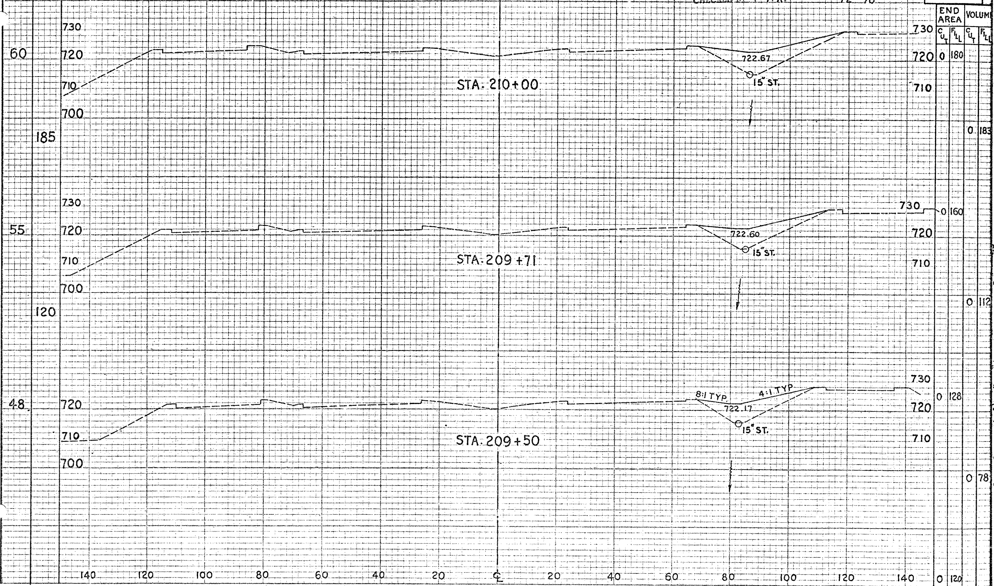
X-SECTIONS STA. 209+50 to STA. 210+00
