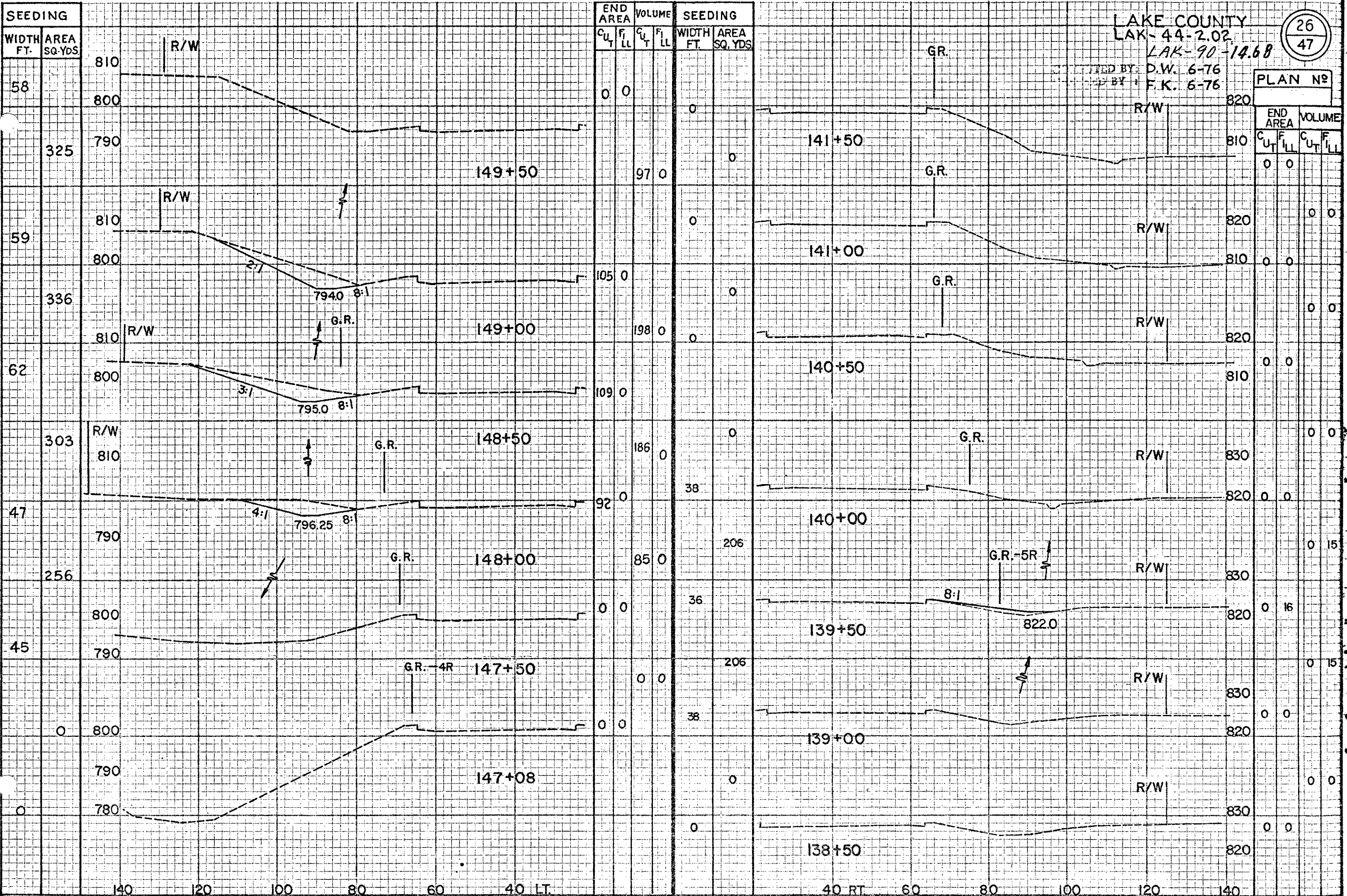
X-SECTIONS STA. 138+50 TO STA. 141+50 (RT.) STA. 147+08 TO STA. 149+50 (LT.)
