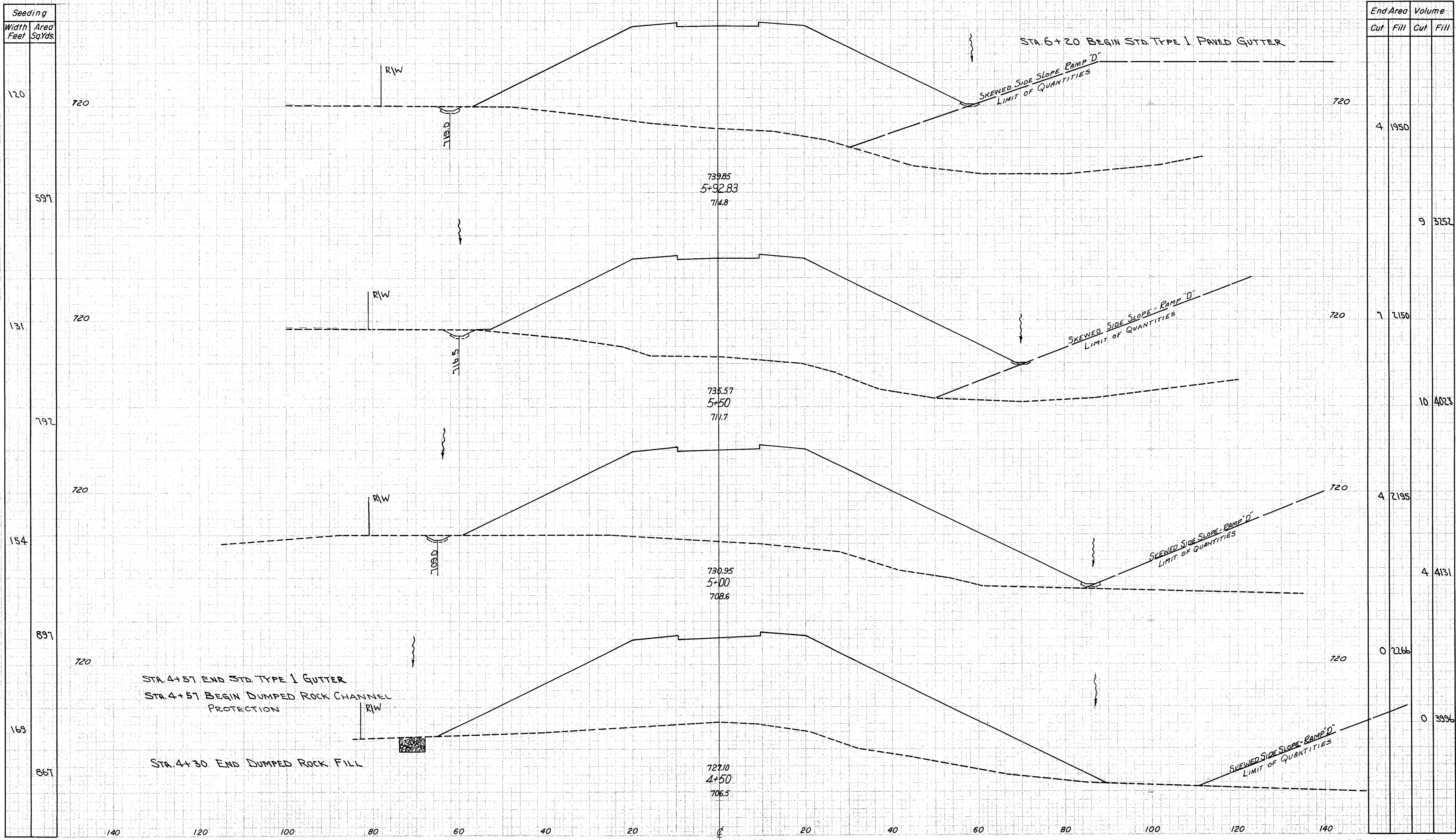
MORLEY ROAD STA. 4+50 TO STA. 5+92.83
