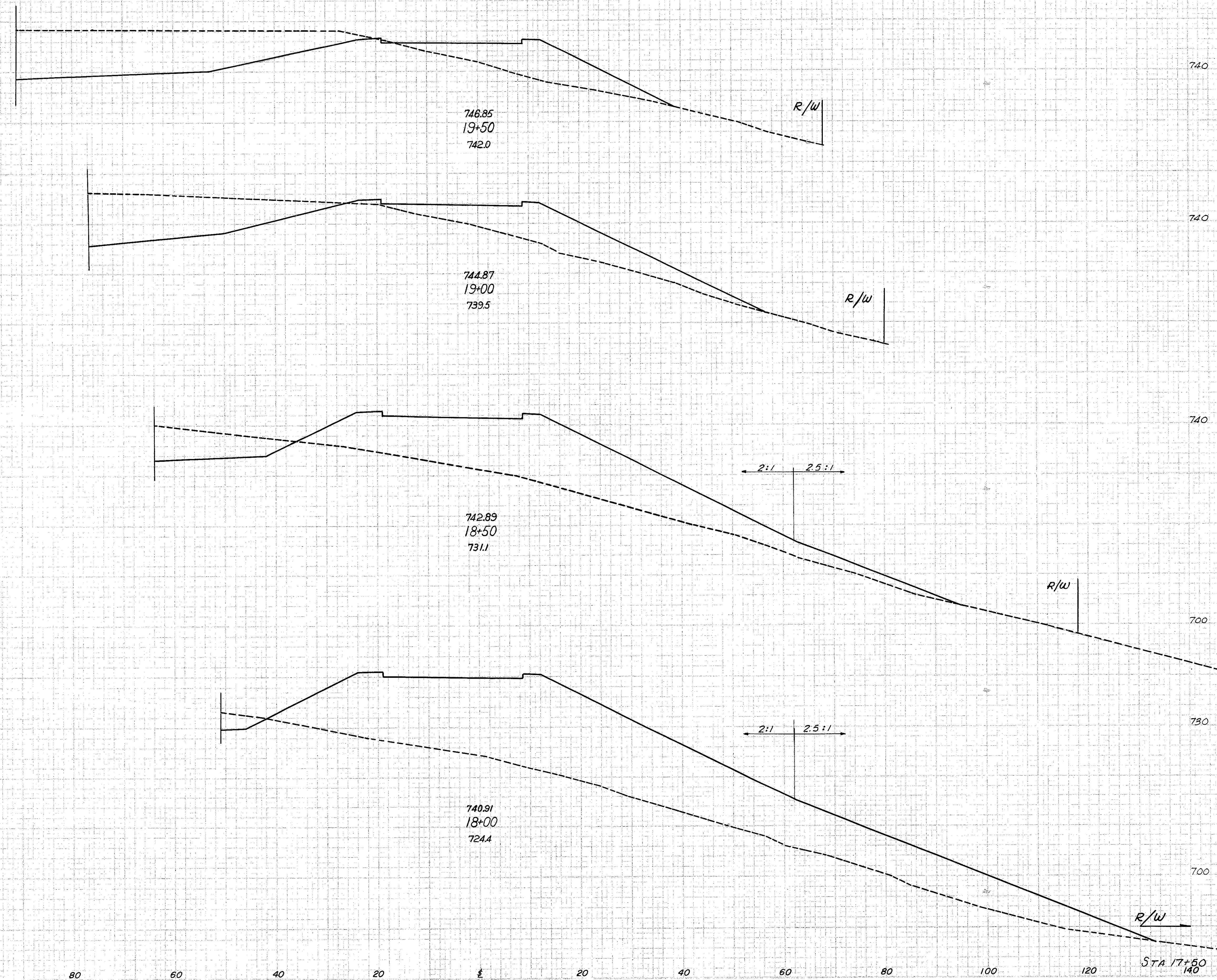
RAMP "C" STA:18+00 TO STA:19+50
