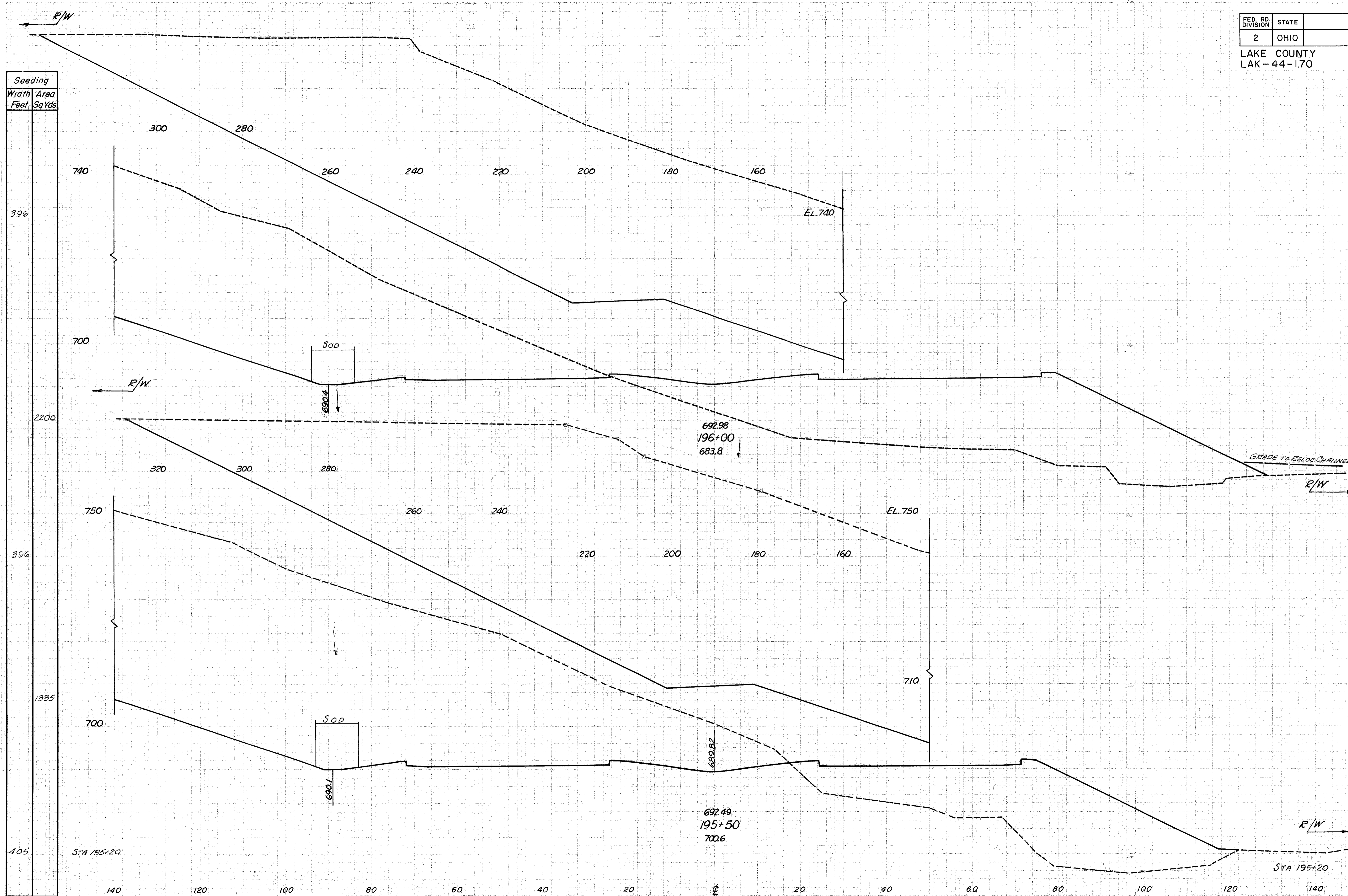
STA. 195+50 TO STA. 196+00
