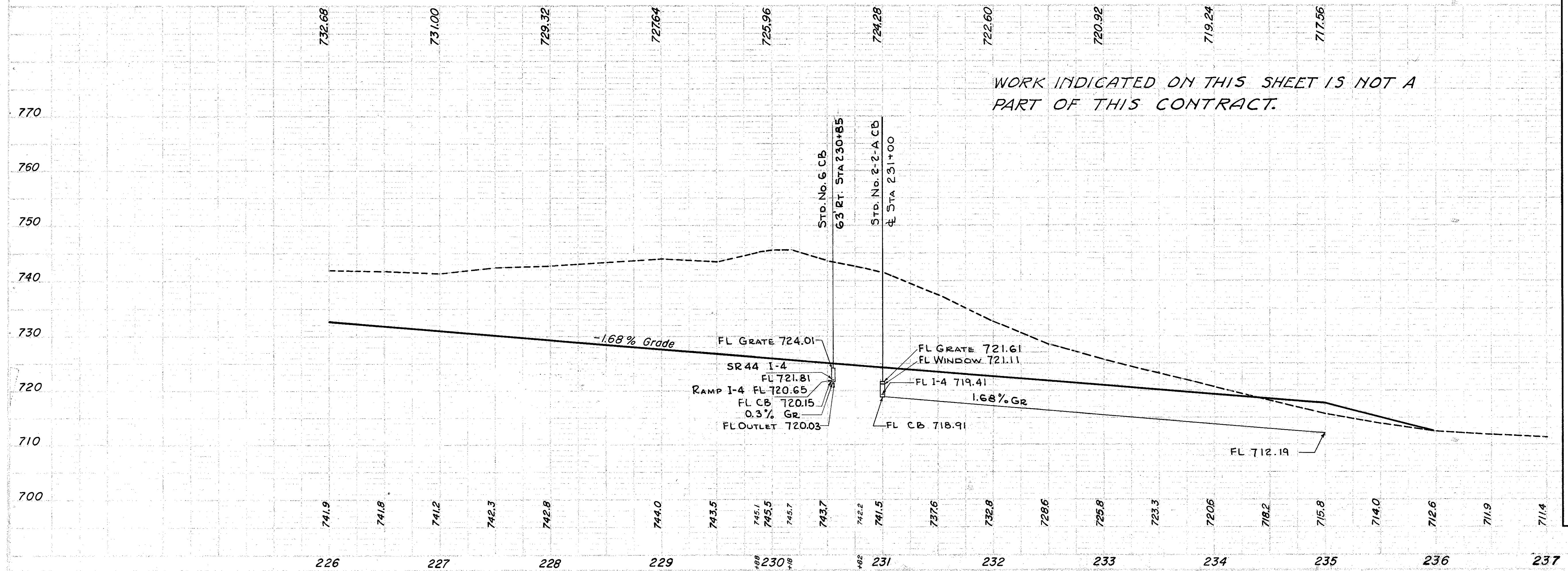
PLAN & PROFILE STA. 226+00 TO STA. 237+00
