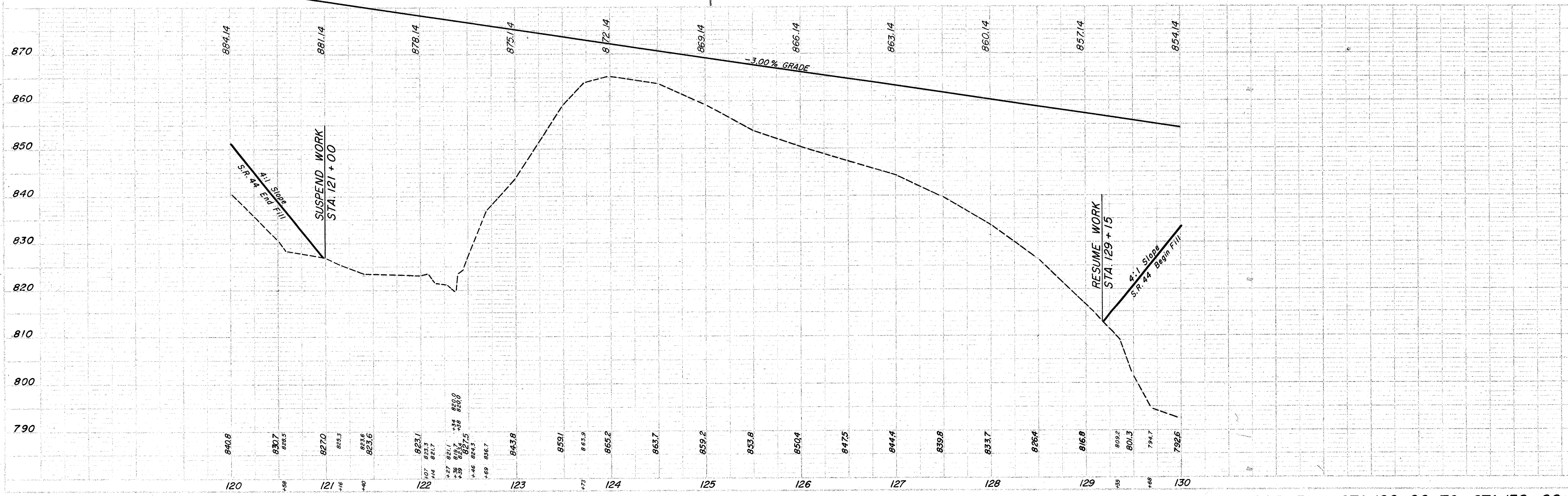
PLAN & PROFILE STA. 120+00 TO STA. 130+00
