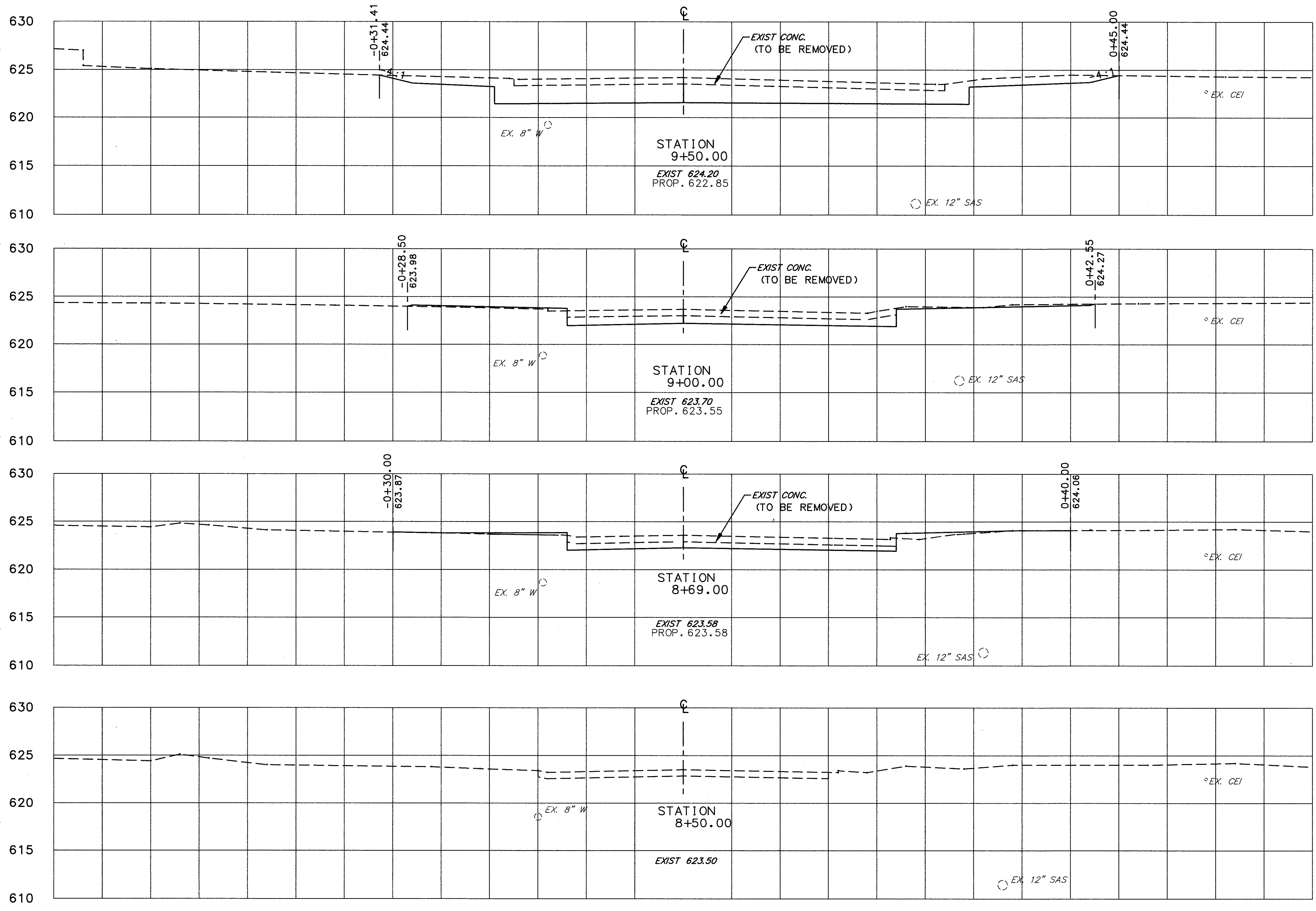
CROSS SECTIONS STA. 8+50 TO STA. 9+50
