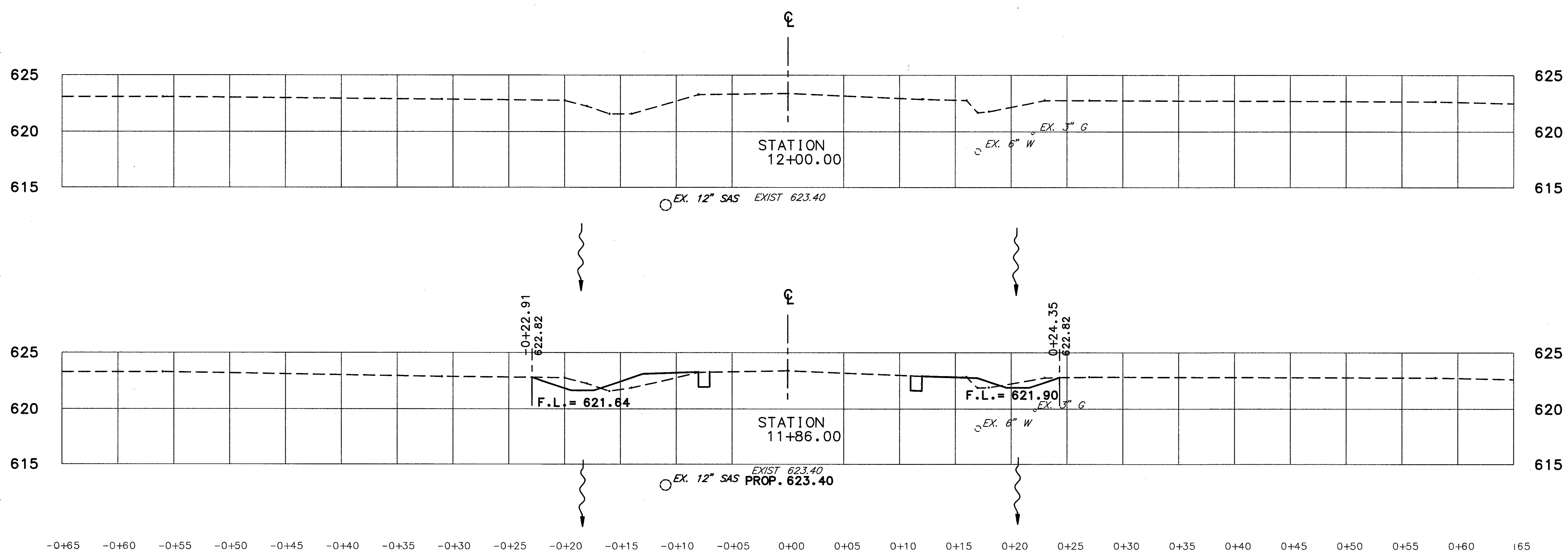
CROSS SECTIONS STA. 11+86 TO STA. 12+00
