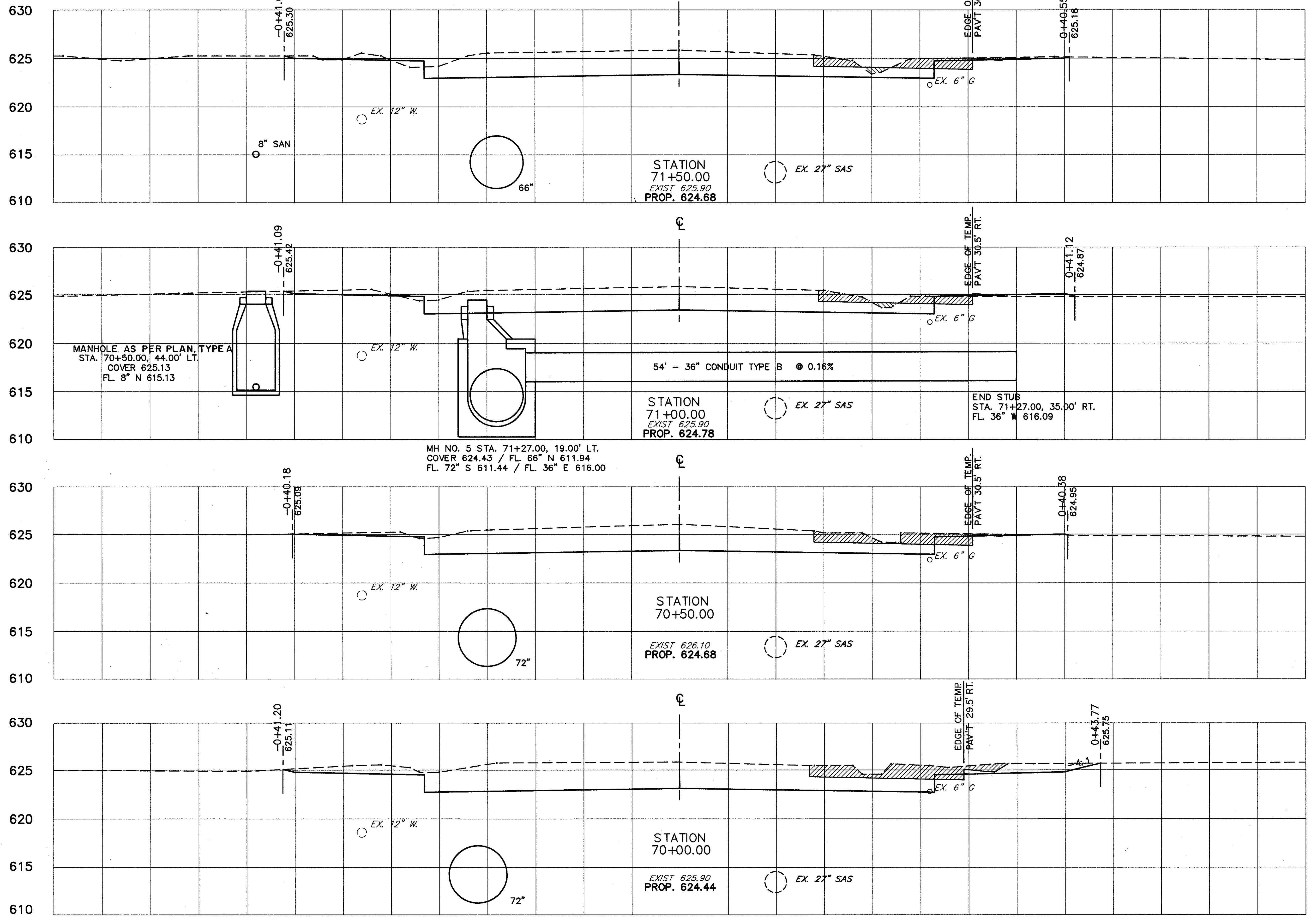
CROSS SECTIONS STA. 70+00 TO STA. 71+50
