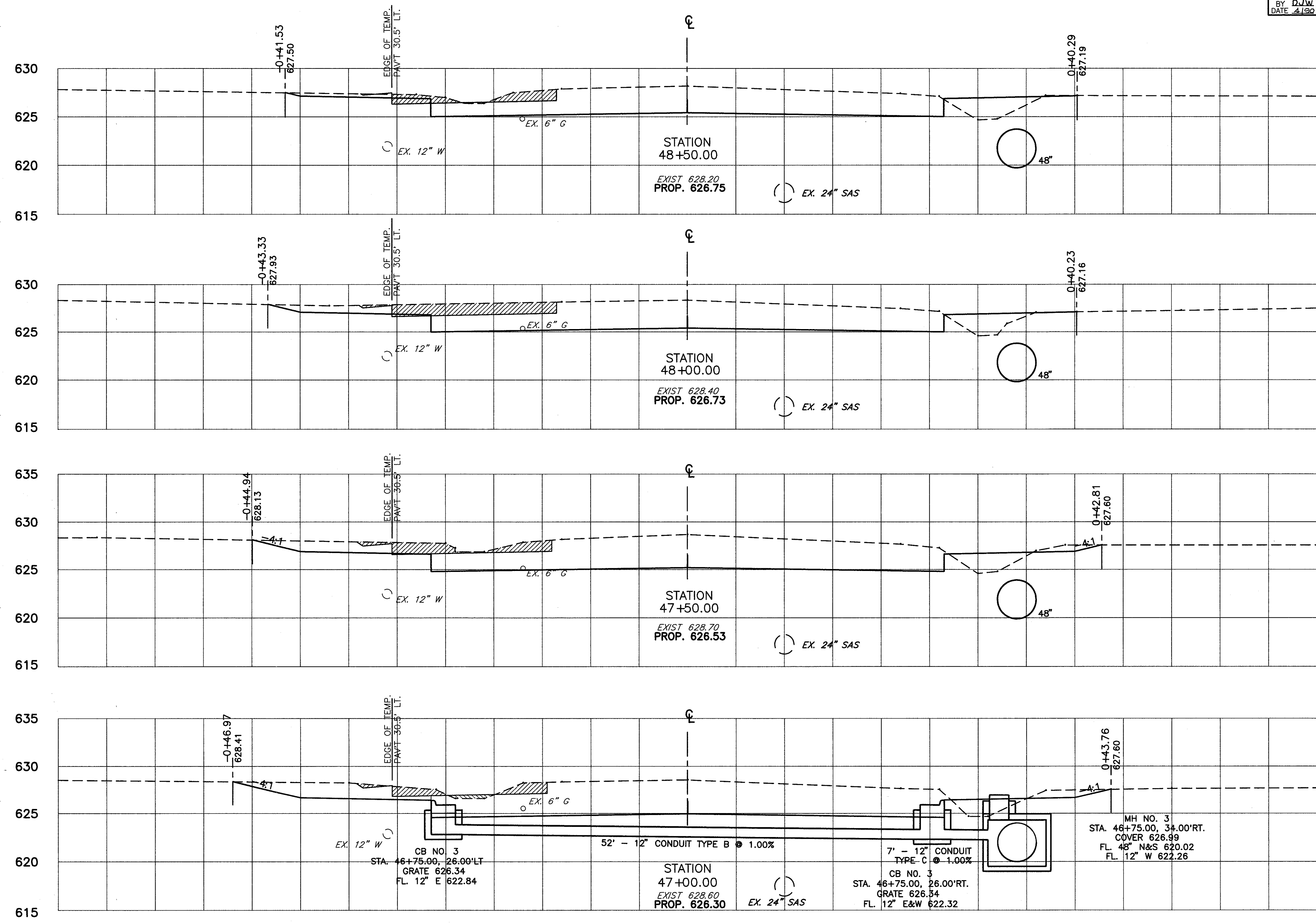
CROSS SECTIONS STA. 47+00 TO STA. 48+50
