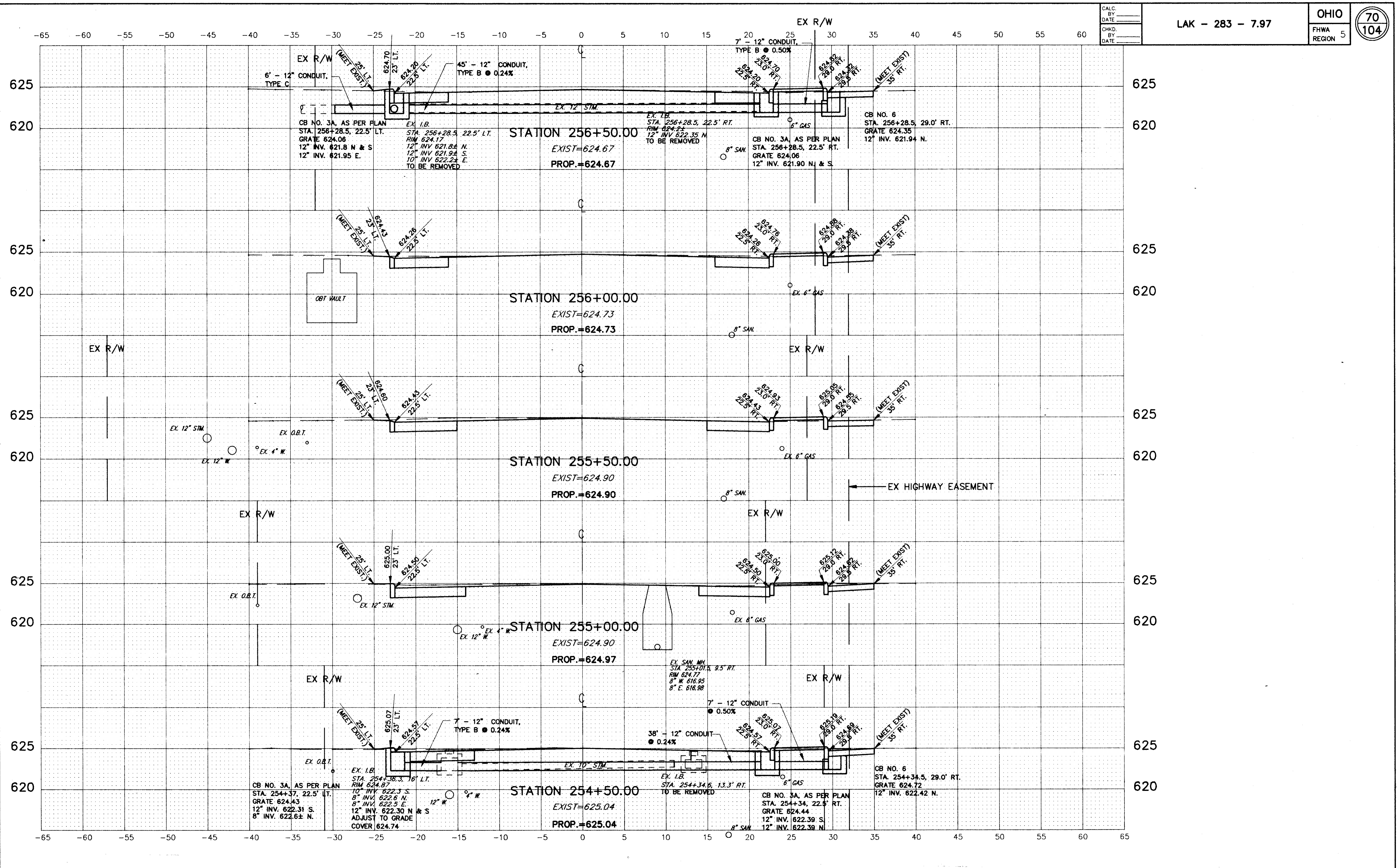
CROSS SECTIONS STA. 254+50 TO STA. 256+50
