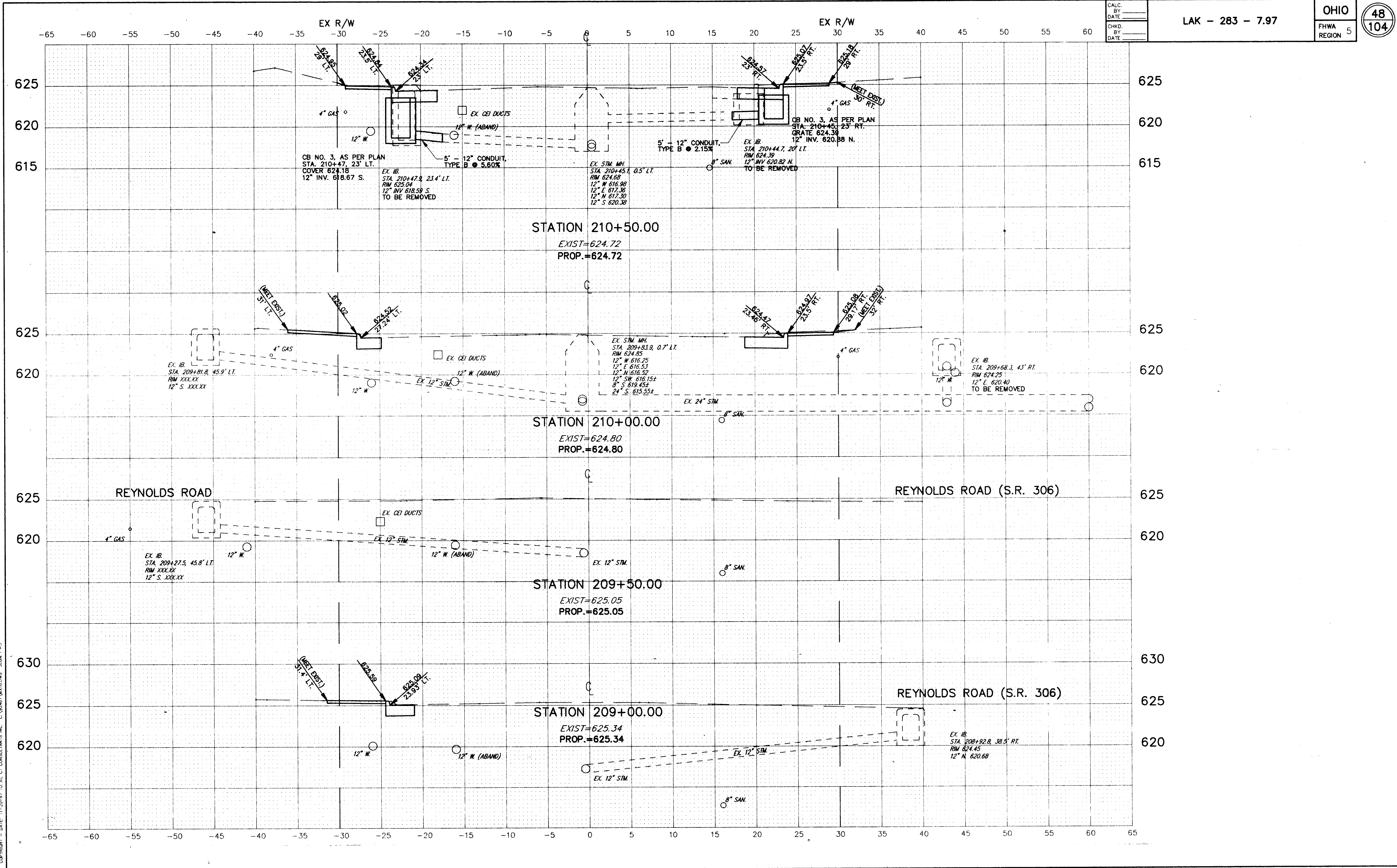
CROSS SECTIONS STA. 209+00 TO STA. 210+50
