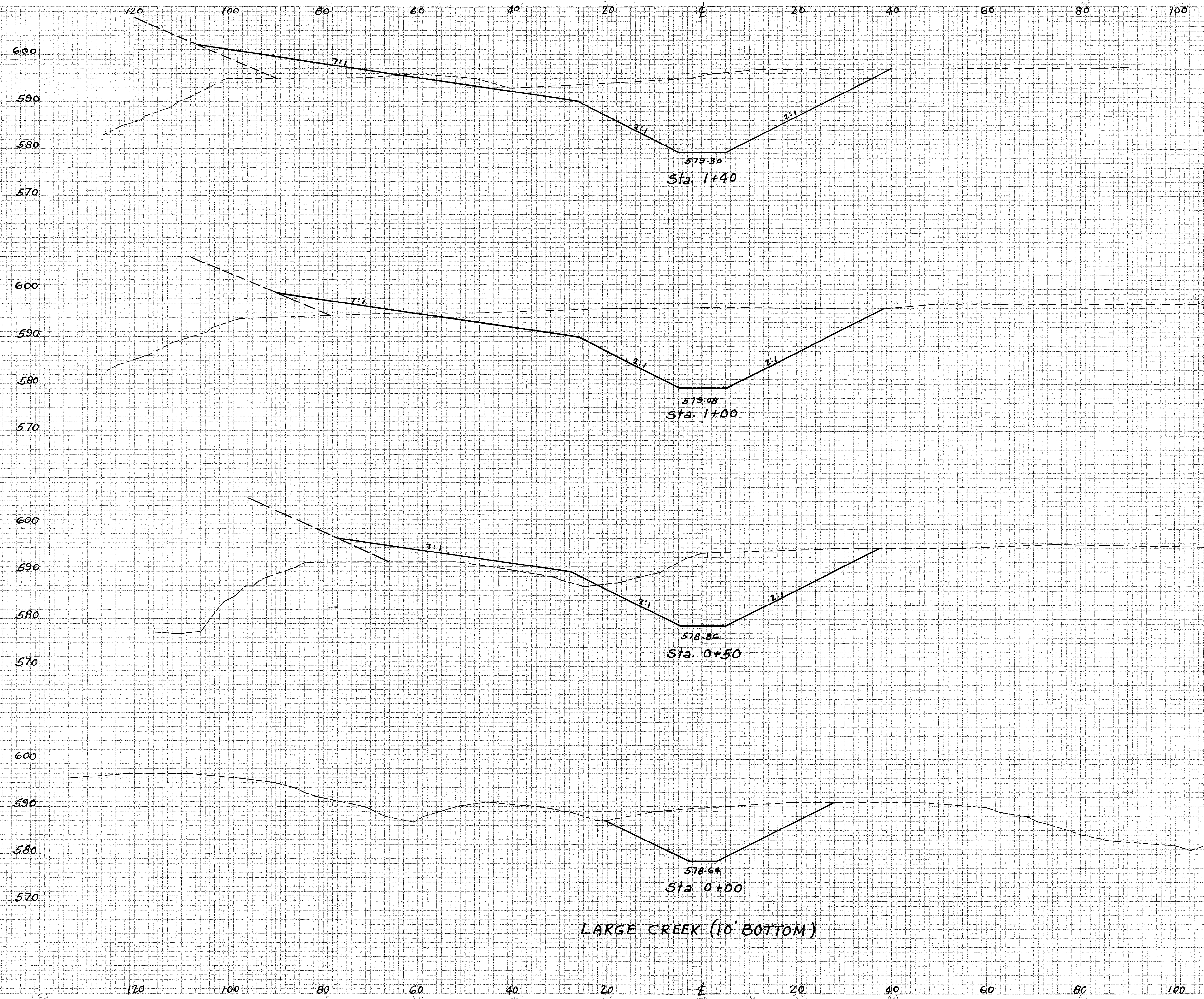
X-SECTIONS STA. 0+00 TO STA. 1+40 (LARGE CREEK)
