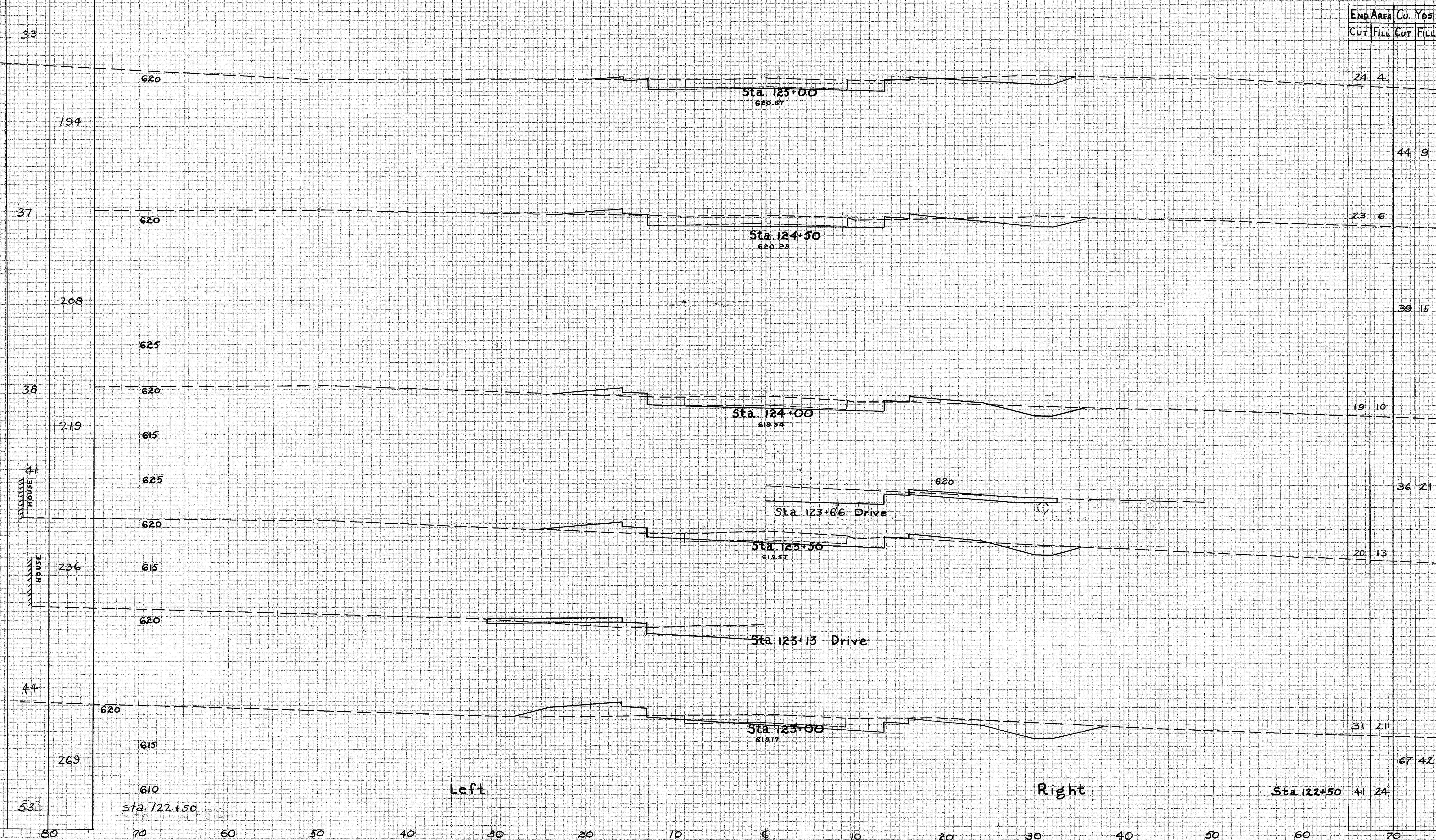
X-SECTIONS STA. 123+00 TO STA. 125+00
