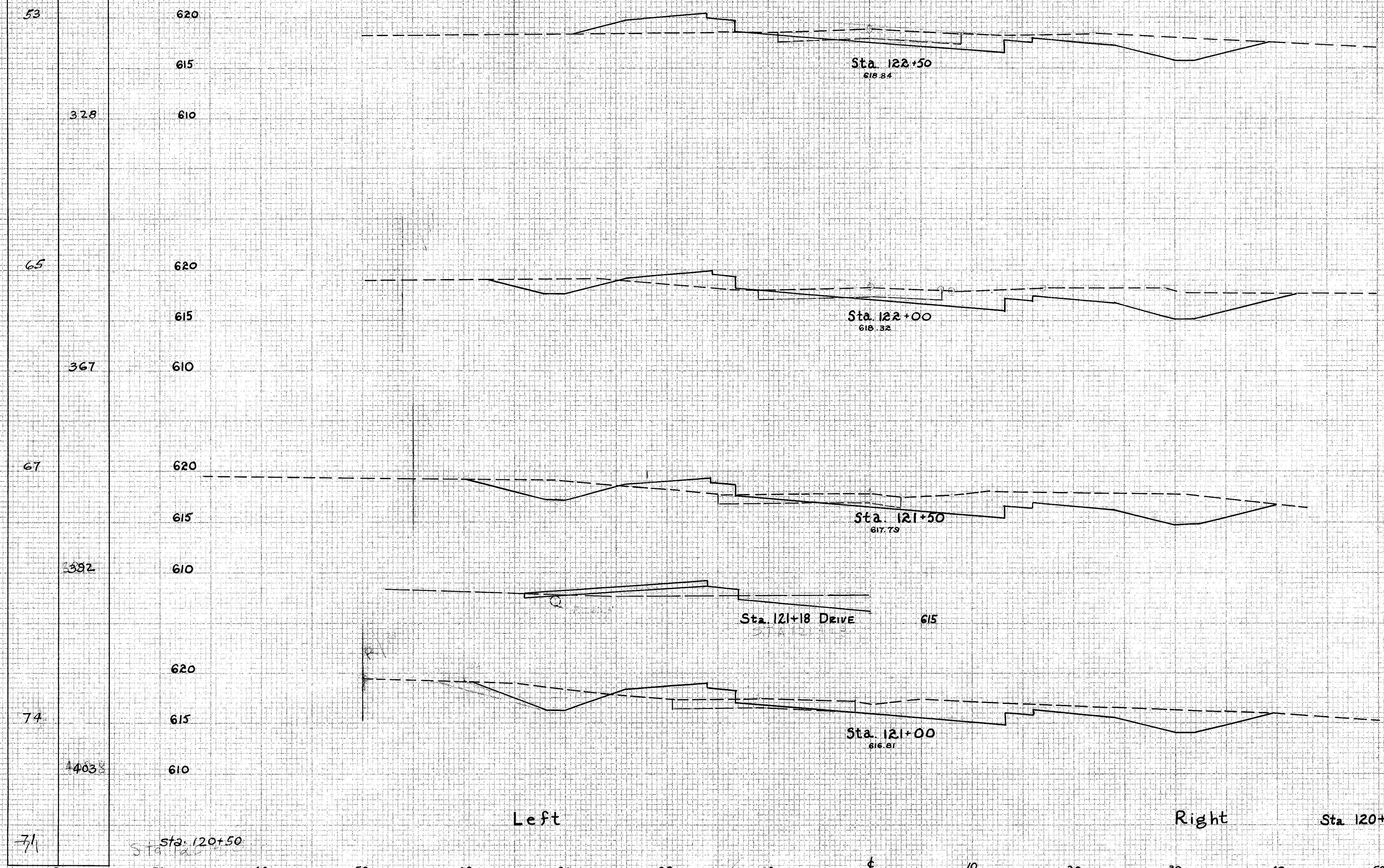
X-SECTIONS STA. 121+00 TO STA. 122+50
