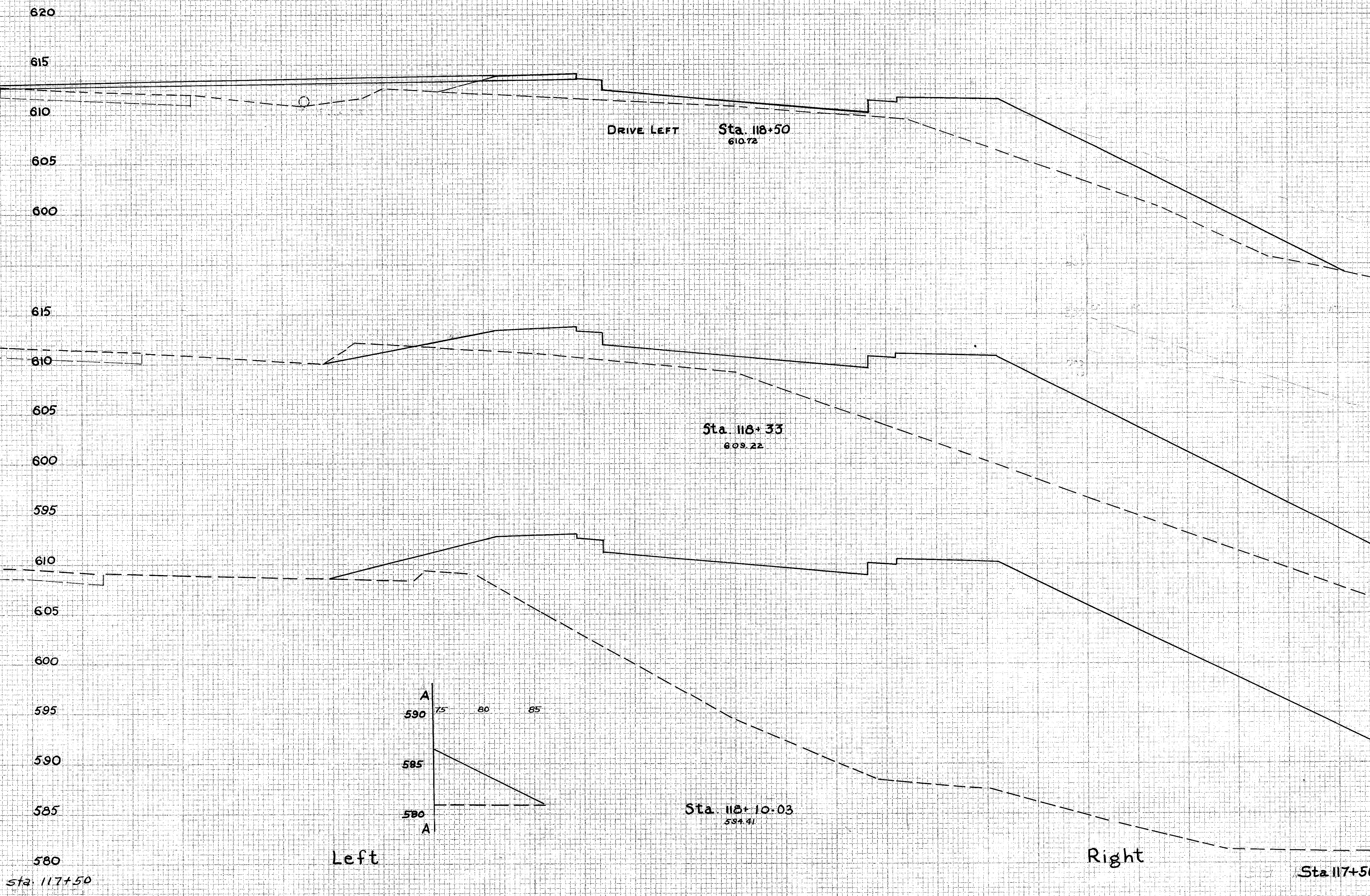
X-SECTIONS STA. 118+00 TO STA. 118+50
