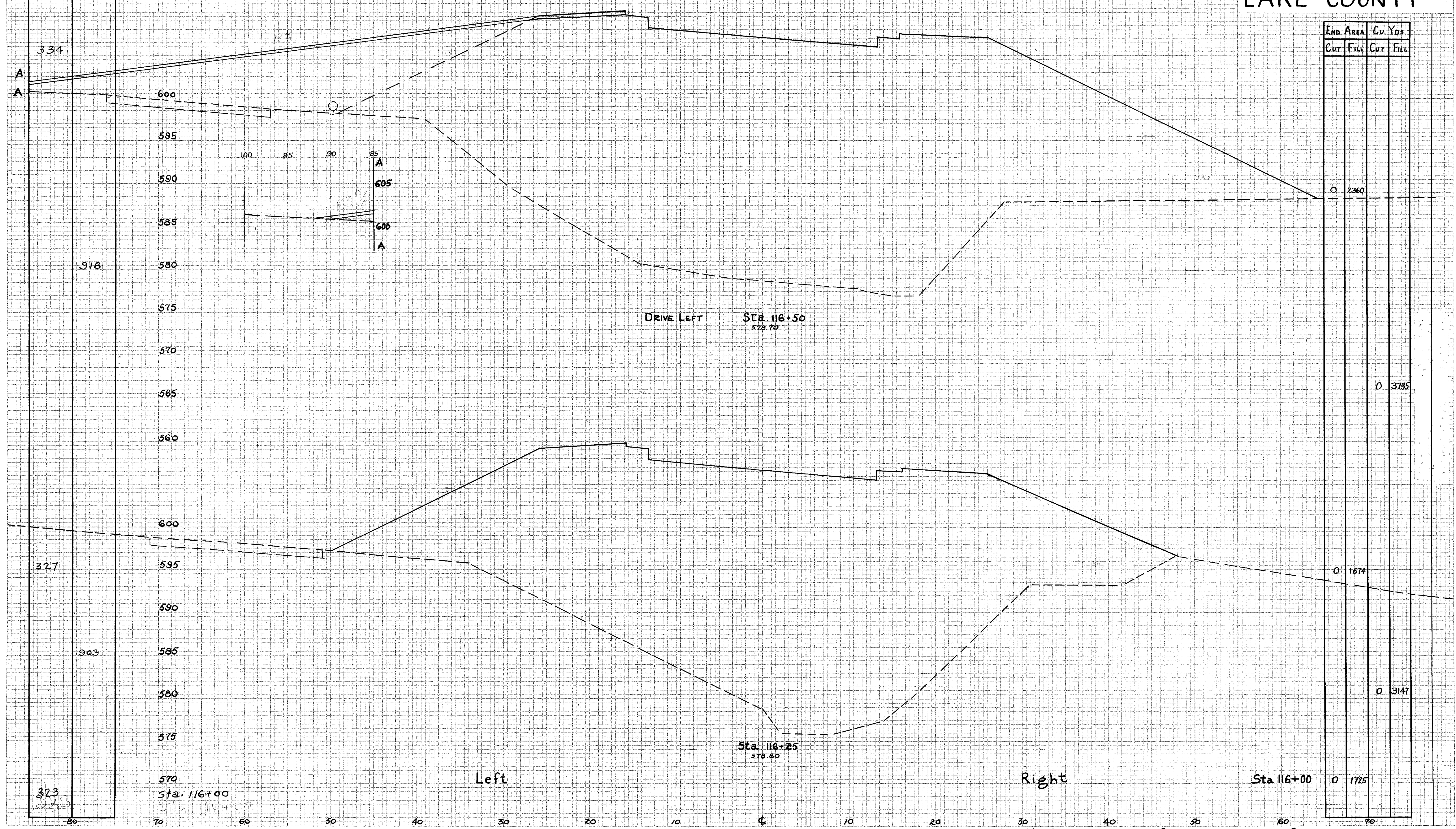
X-SECTIONS STA. 116+25 TO STA. 116+50
