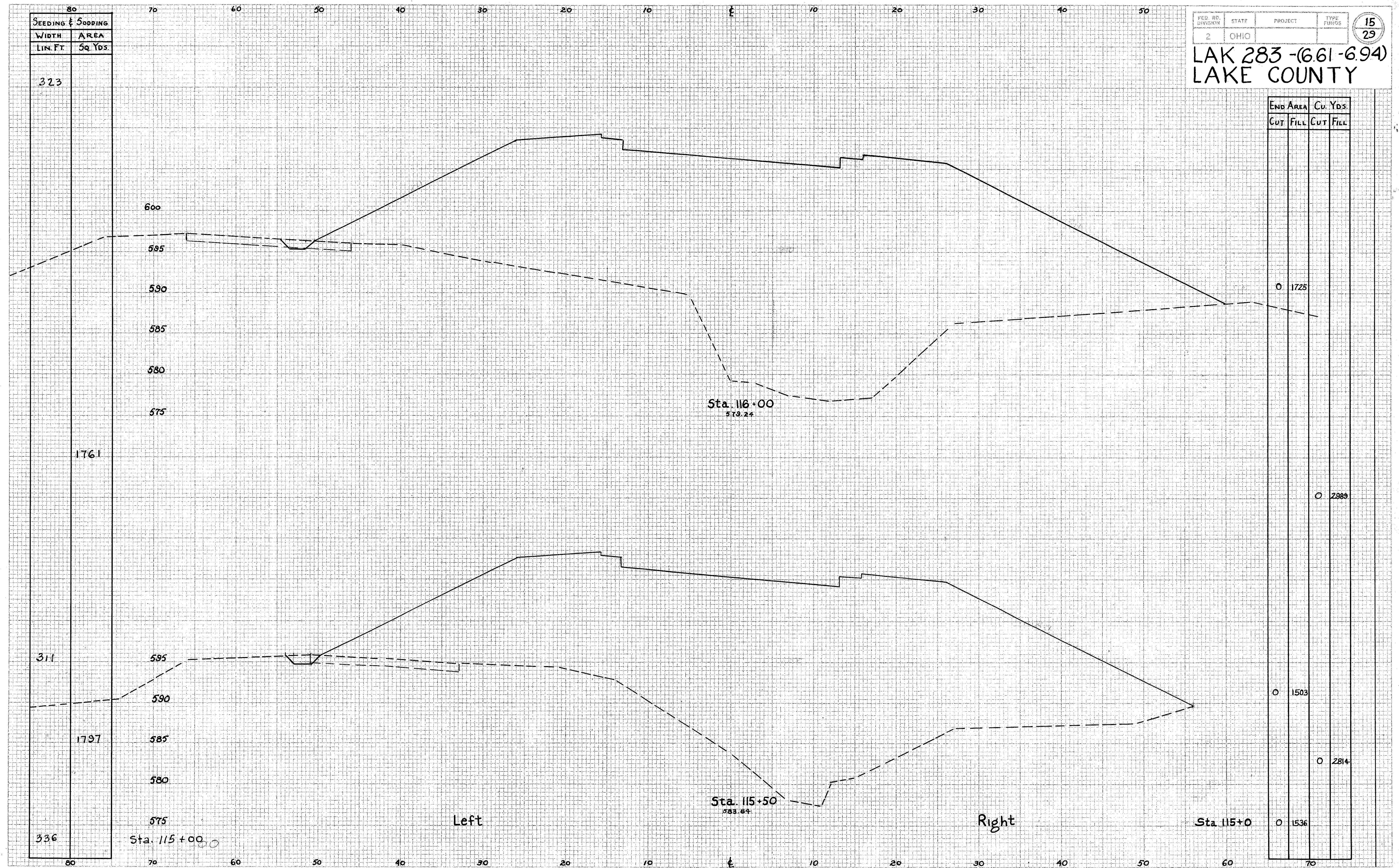
X-SECTIONS STA. 115+50 TO STA. 116+00
