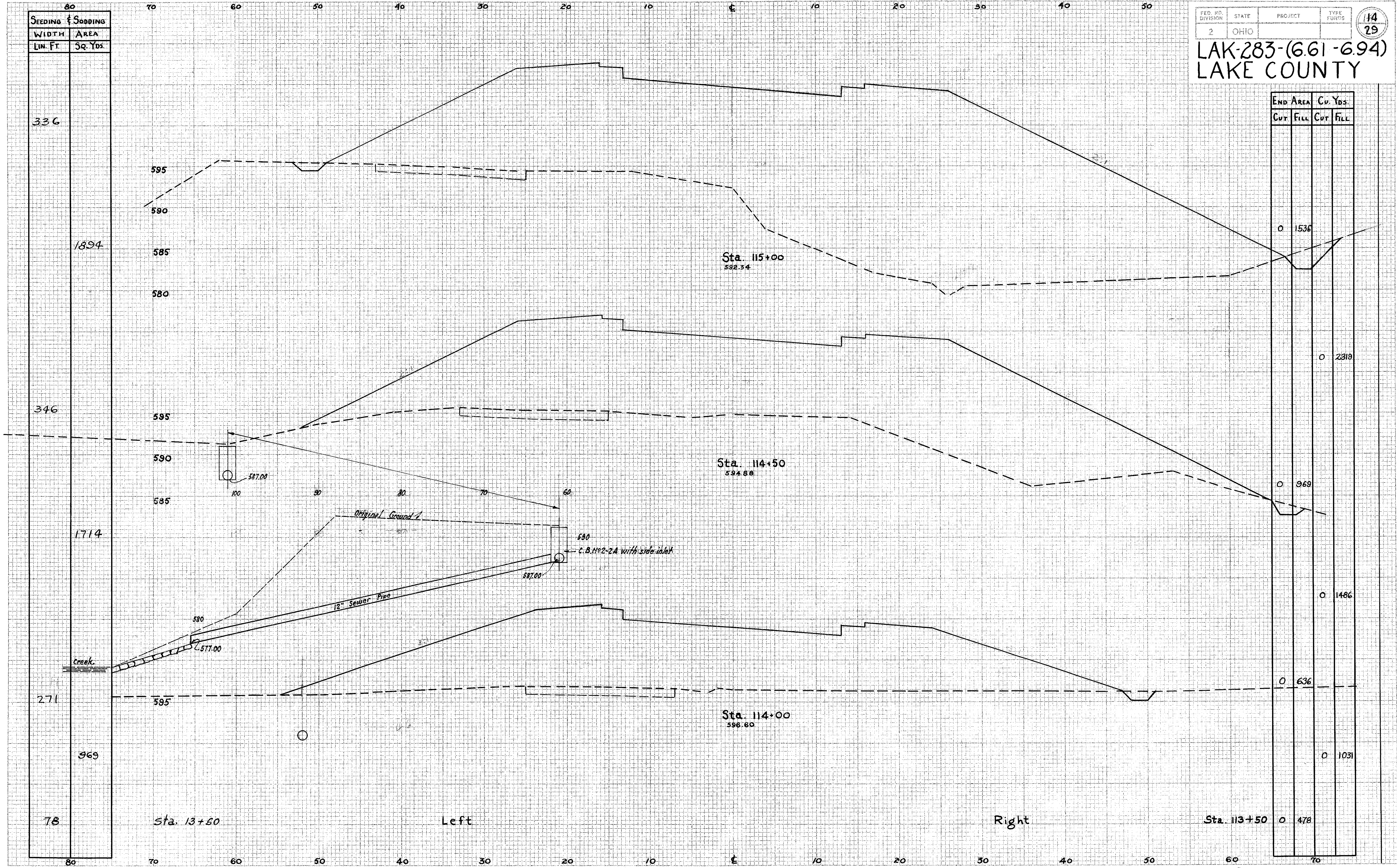
X-SECTIONS STA. 114+00 TO STA. 115+00
