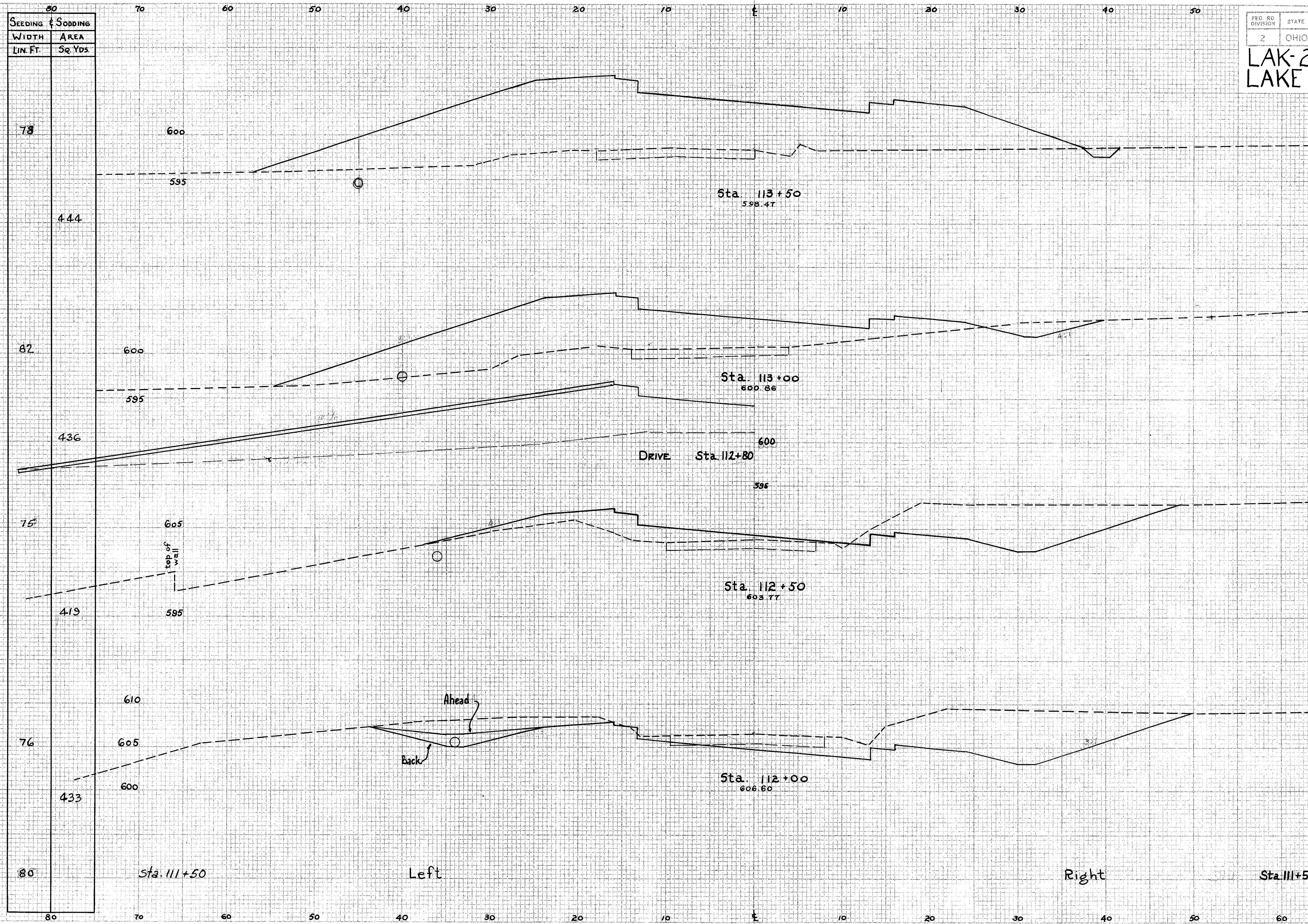
X-SECTIONS STA. 112+00 TO STA. 113+50
