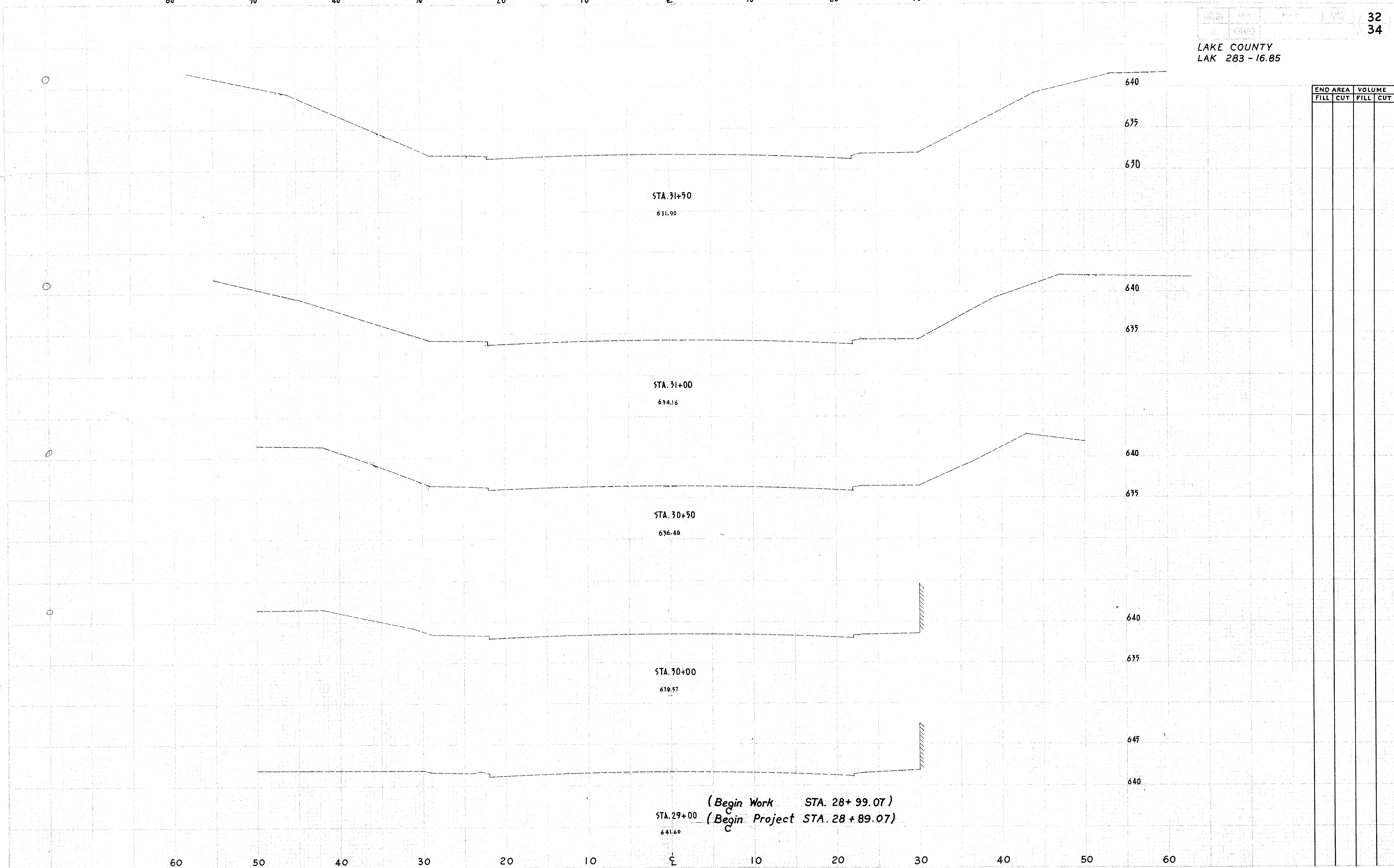
CROSS SECTIONS ... S.R. 283 ... STA. 29+00 to STA. 31+50
