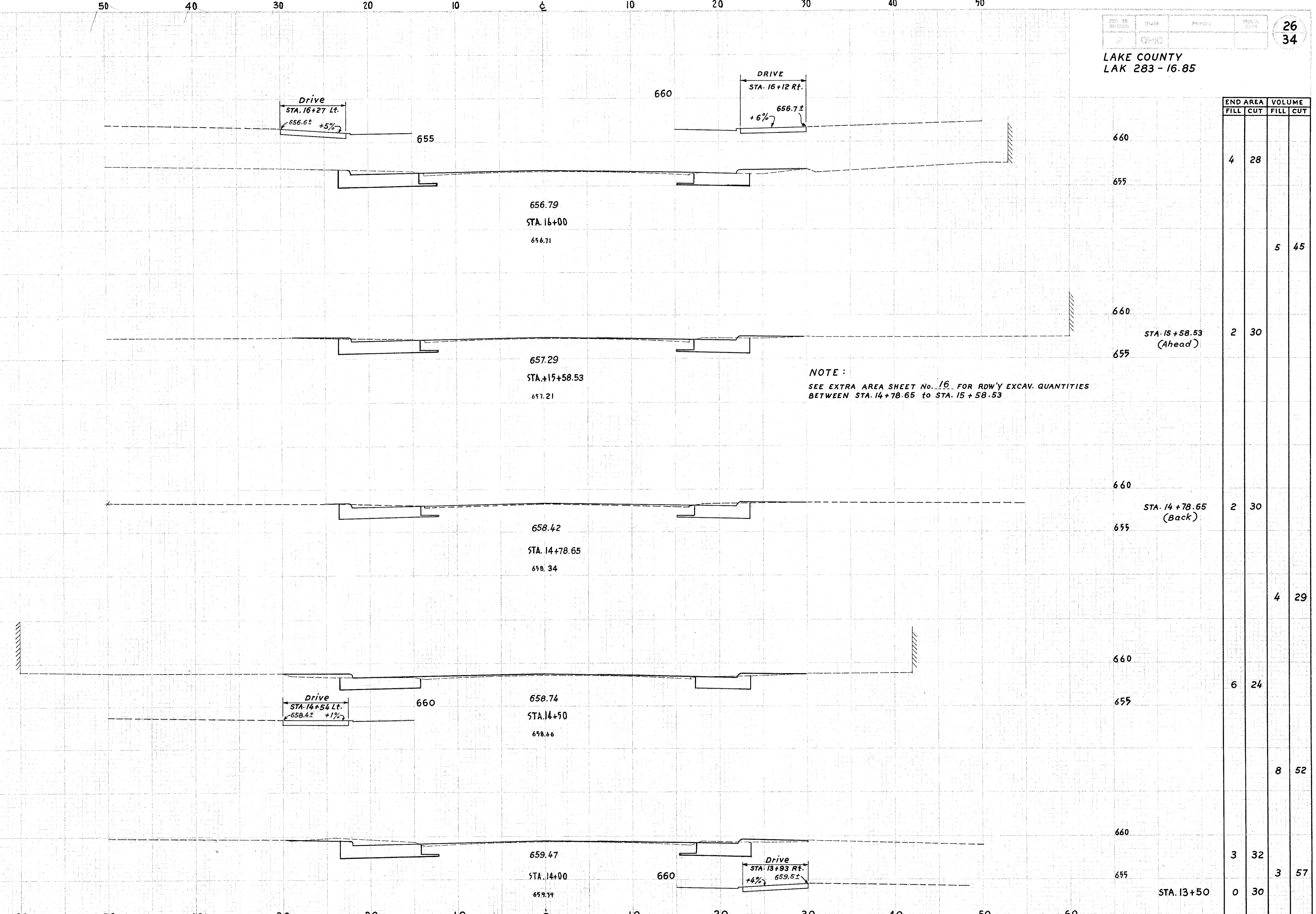
CROSS SECTIONS ... S.R. 283 ... STA. 14+00 to STA. 16+00
