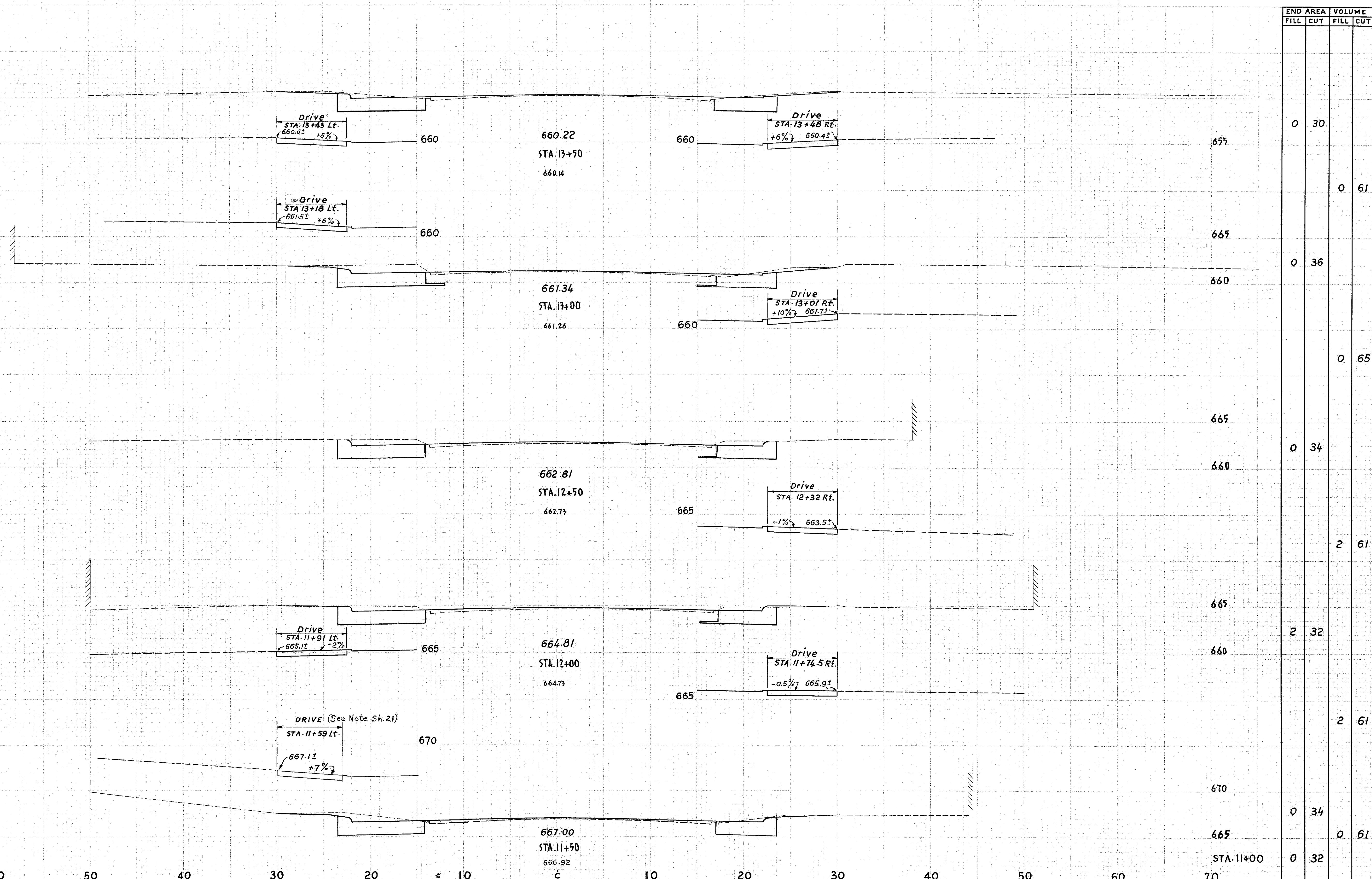
CROSS SECTIONS ... S.R. 283 ... STA. 11+50 to STA. 13+50
