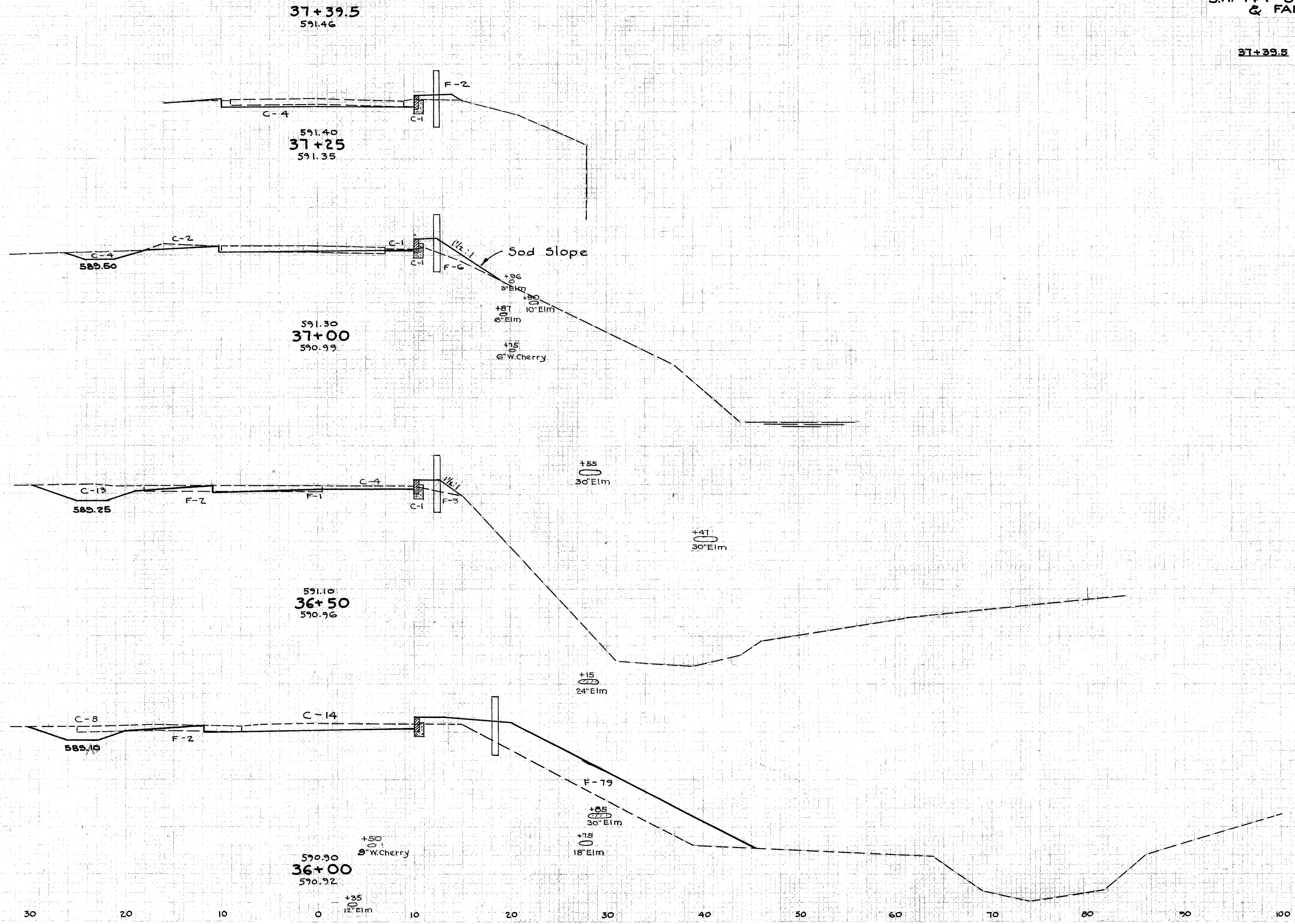
CROSS SECTIONS STA. 36+00 To STA. 37+39.5
