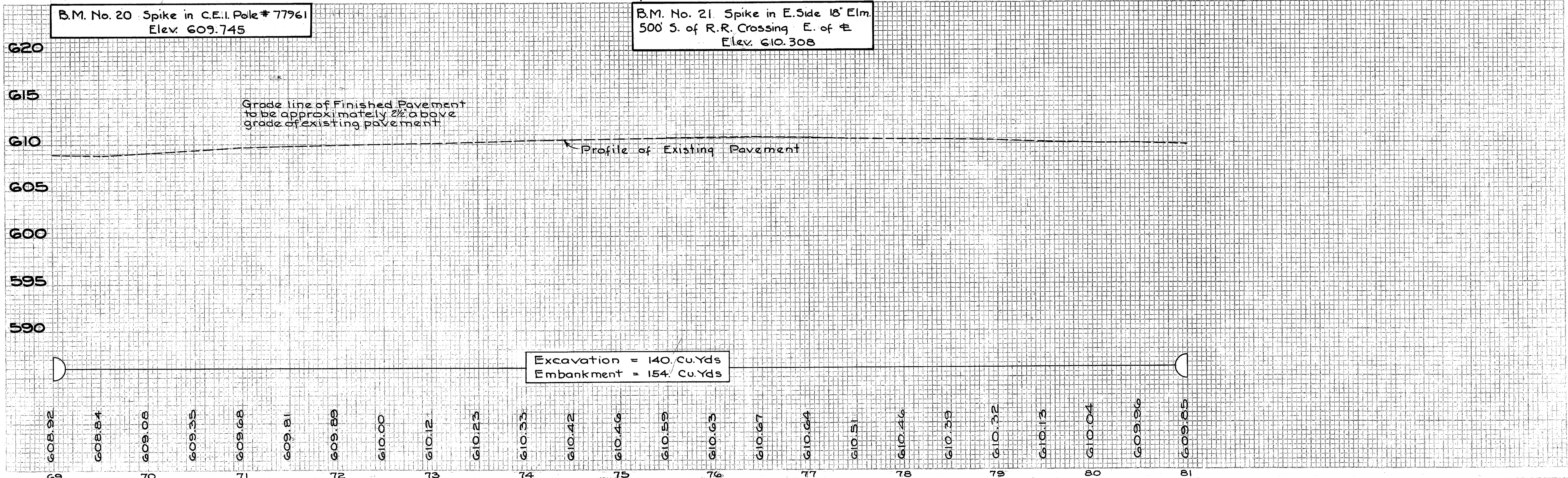
PLAN & PROFILE STA. 69+00 TO STA. 81+00
