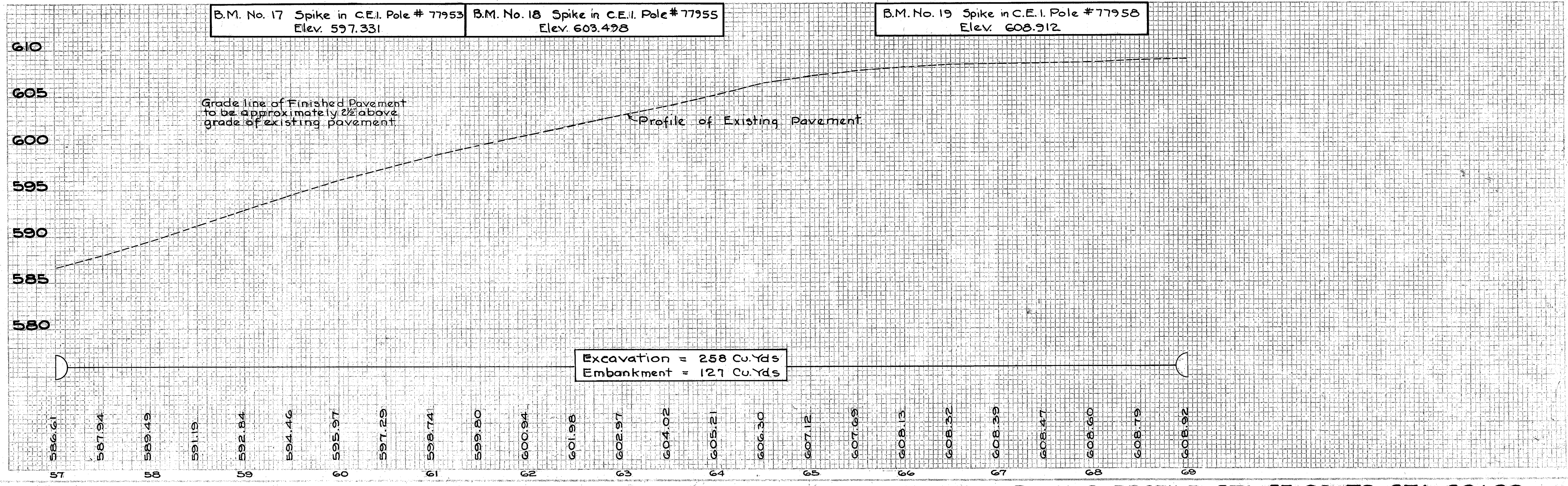
PLAN & PROFILE STA. 57+00 TO STA. 69+00
