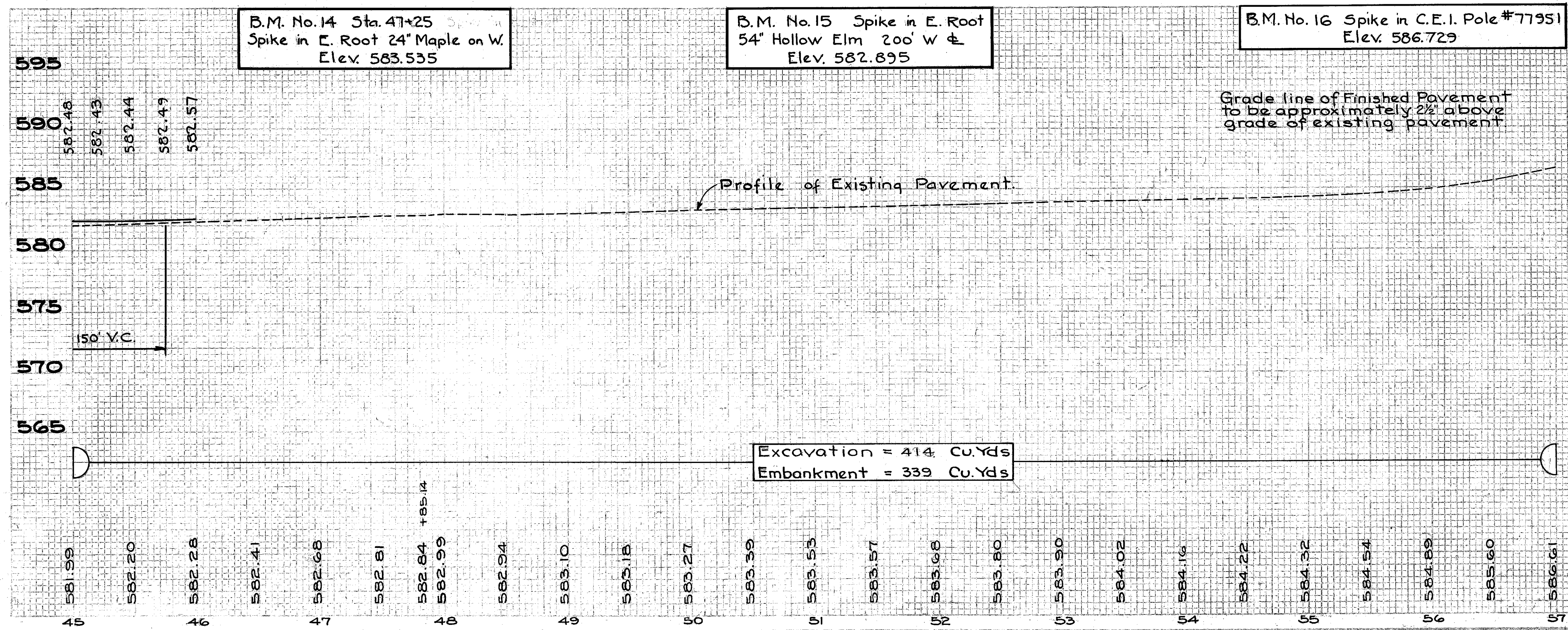
PLAN & PROFILE STA. 45+00 TO STA. 57+00
