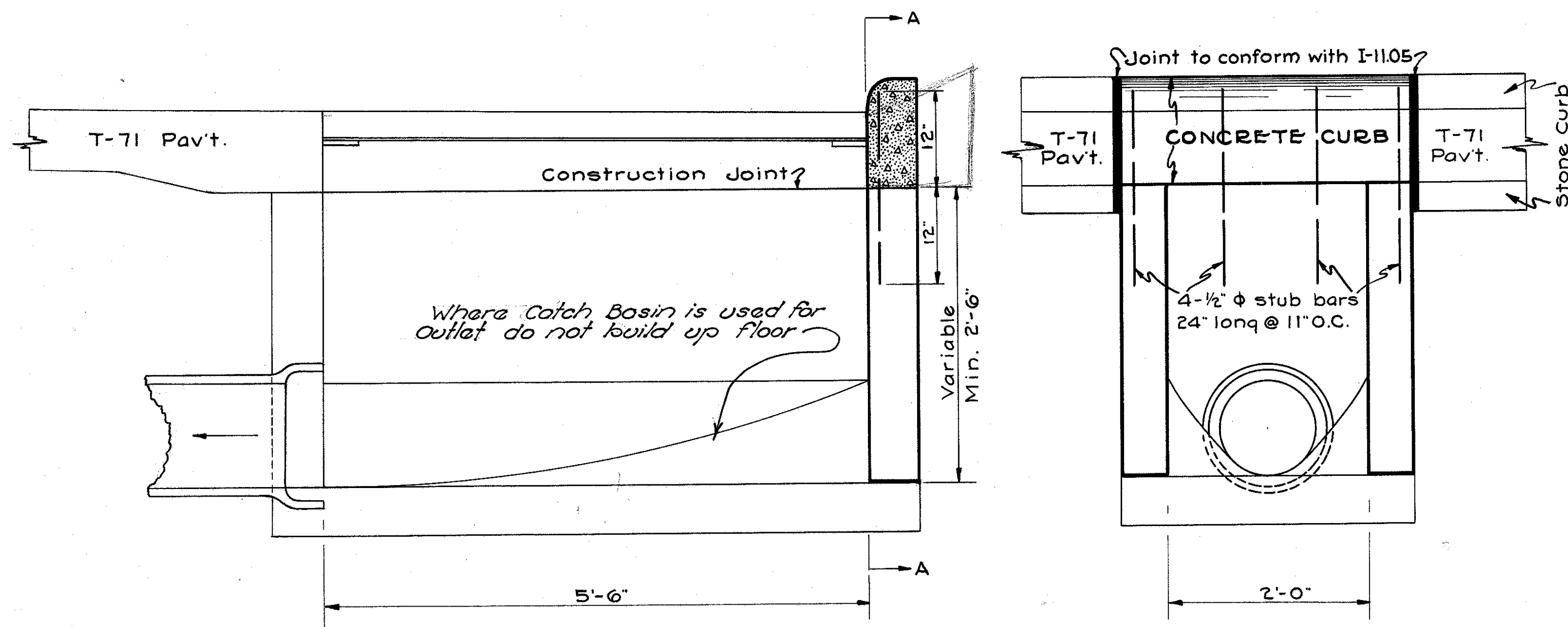
SECTION A-A
