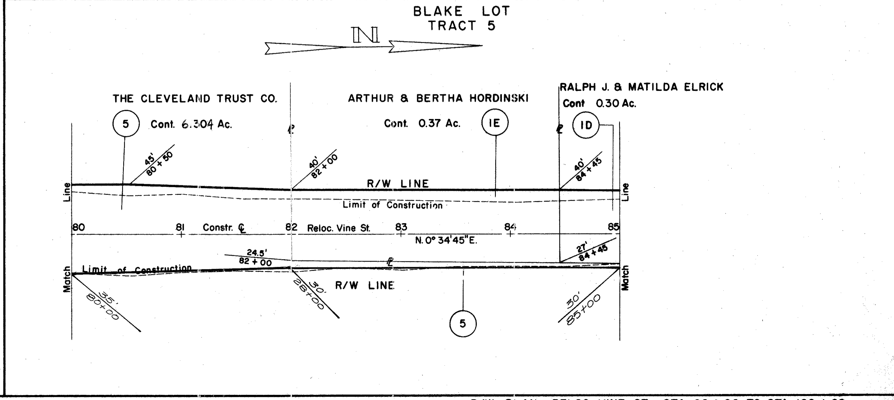
R/W PLAN RELOC. VINE ST. STA. 80+00 TO STA. 100+00
