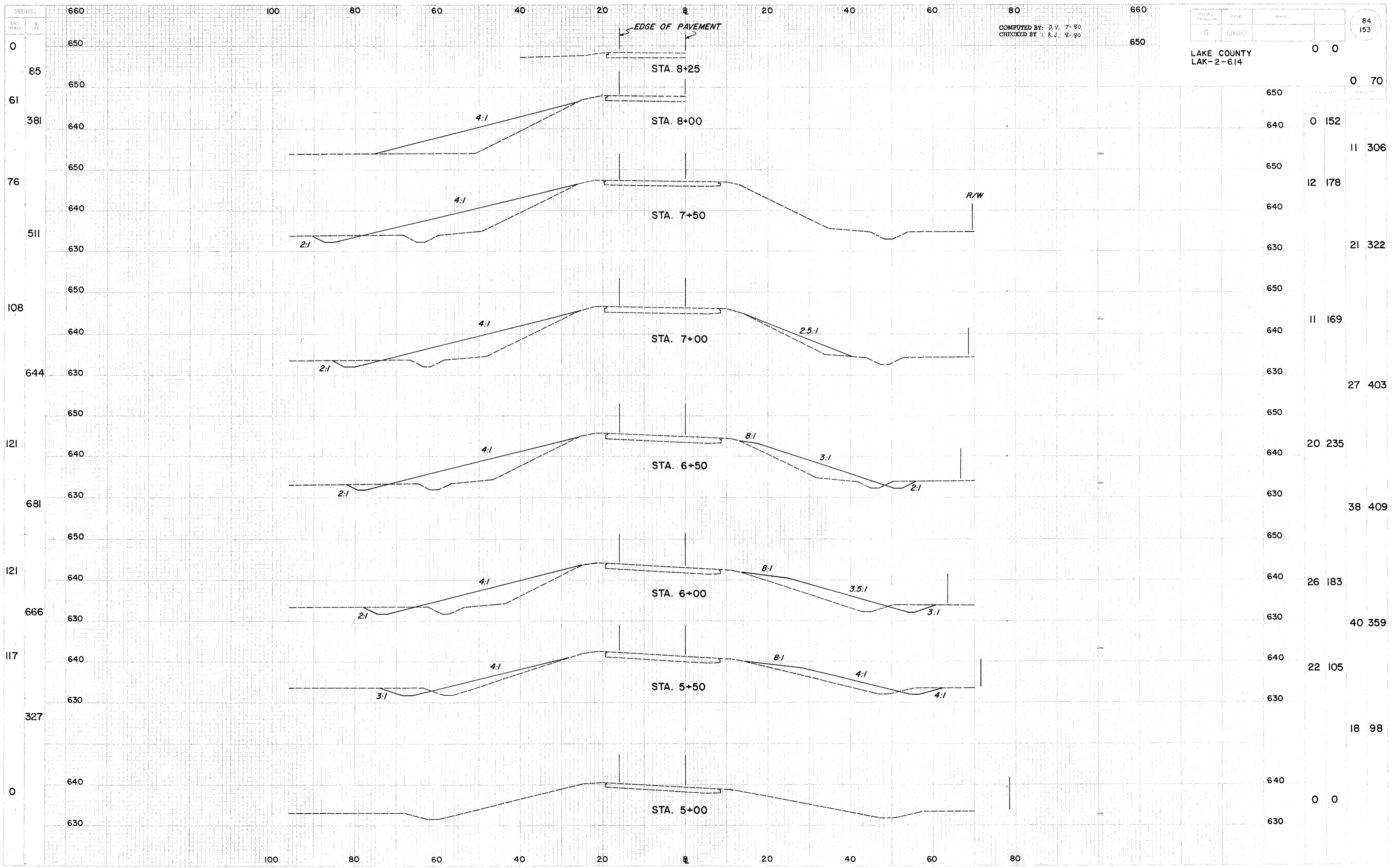
RAMP F-6 STA. 5+00 TO STA. 8+25
