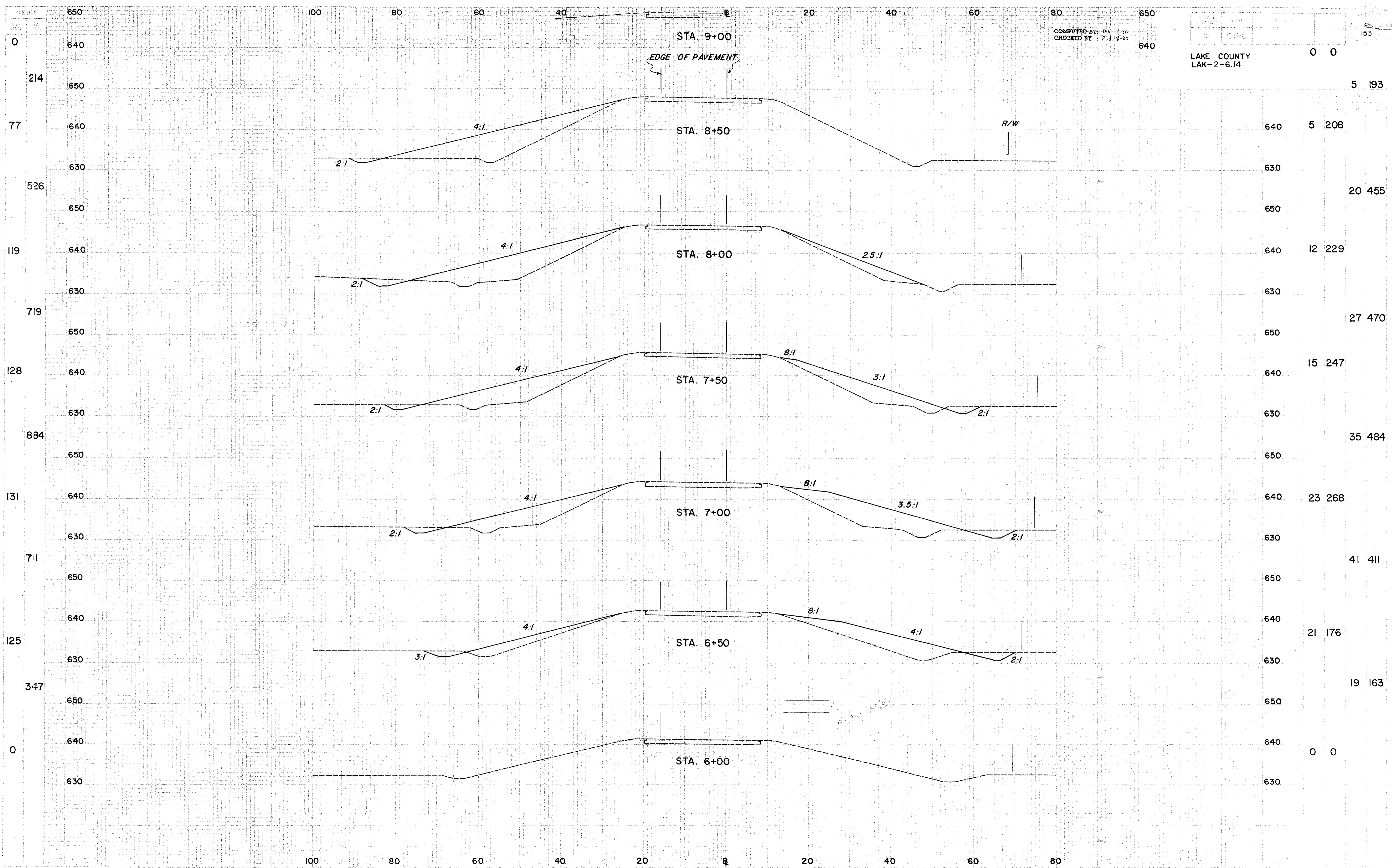
RAMP F-3 STA. 6+00 TO STA. 9+00
