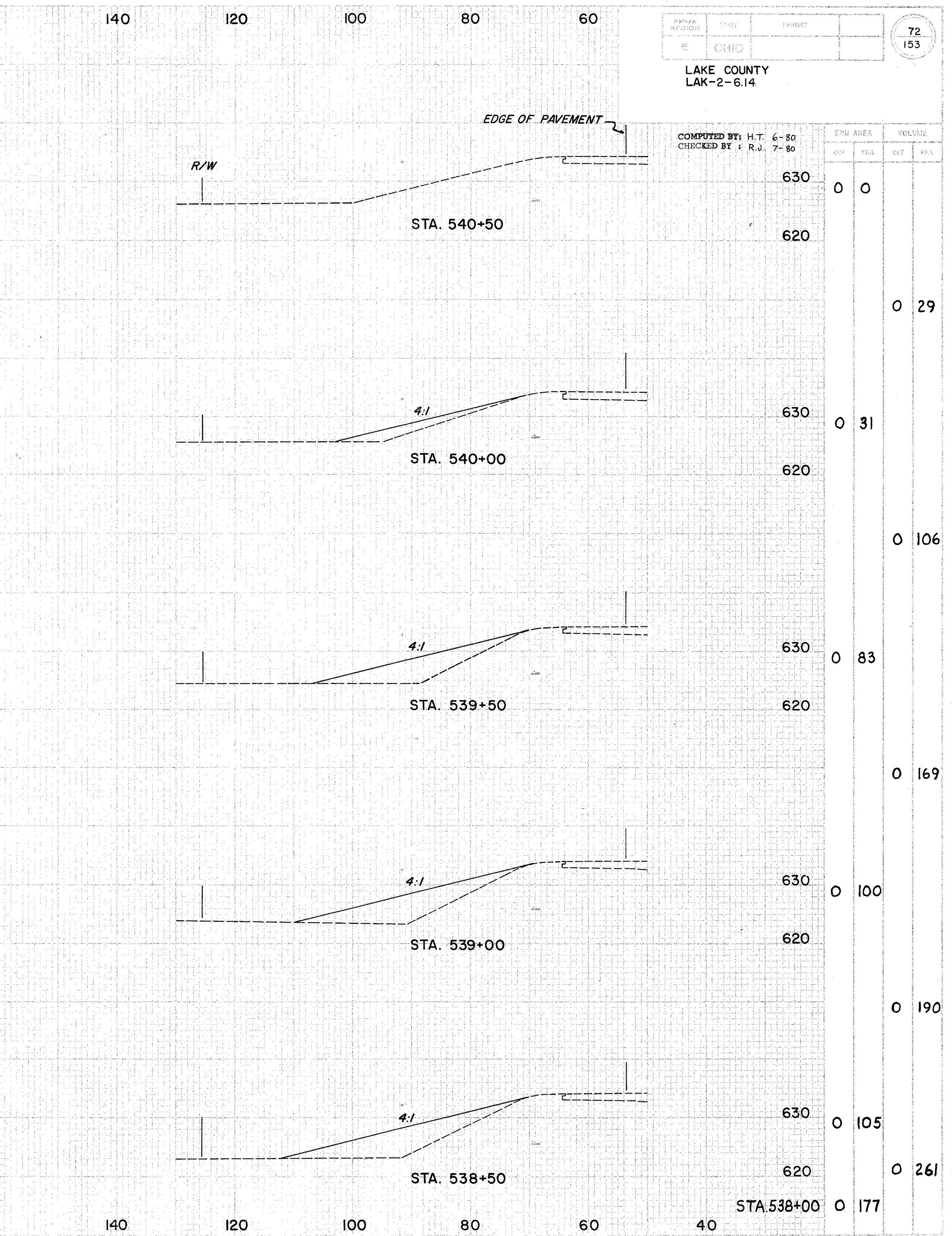
STA. 536+00 TO STA. 540+50 LT.
