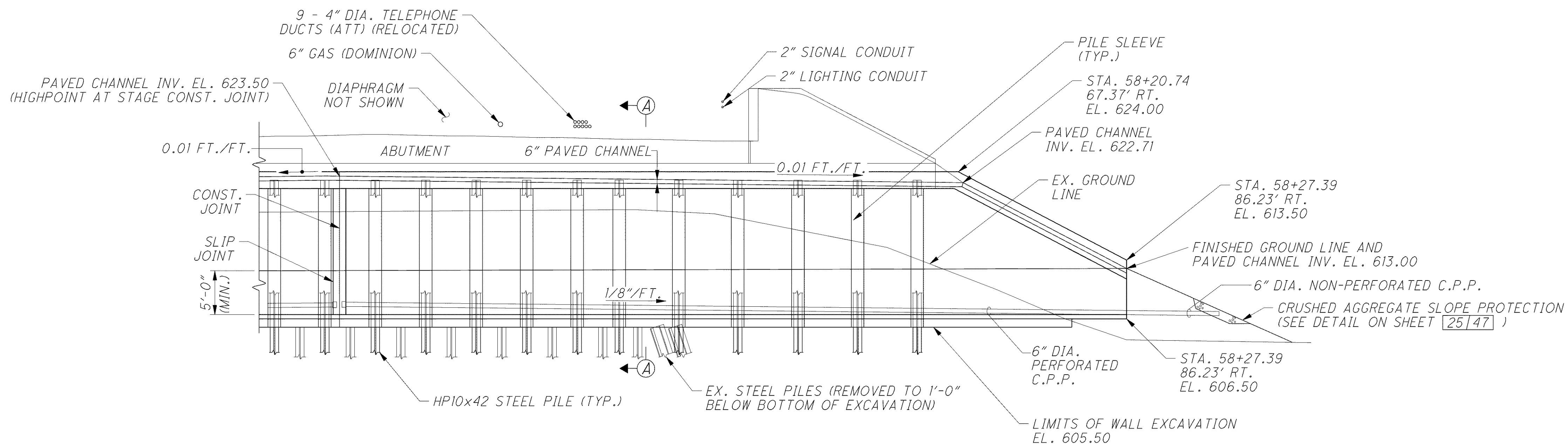
ELEVATION
