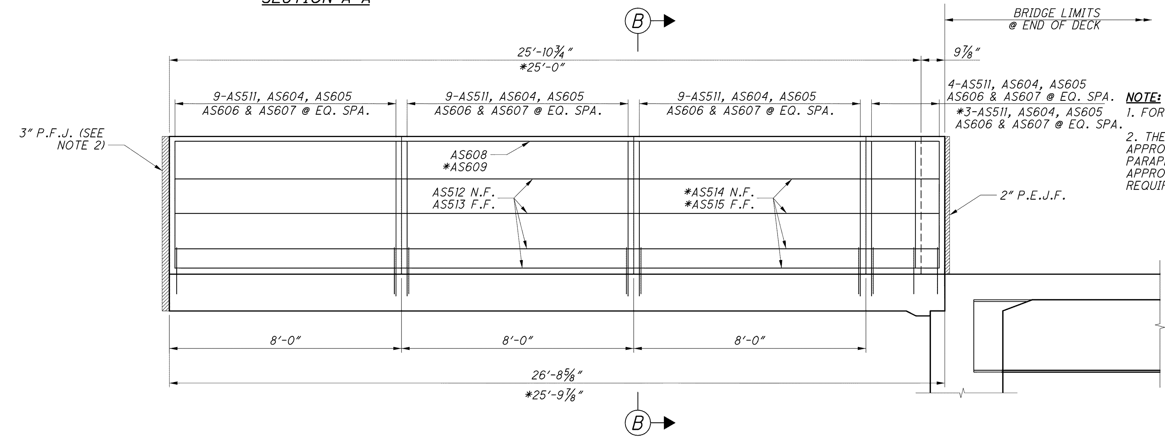
SECTION A-A
