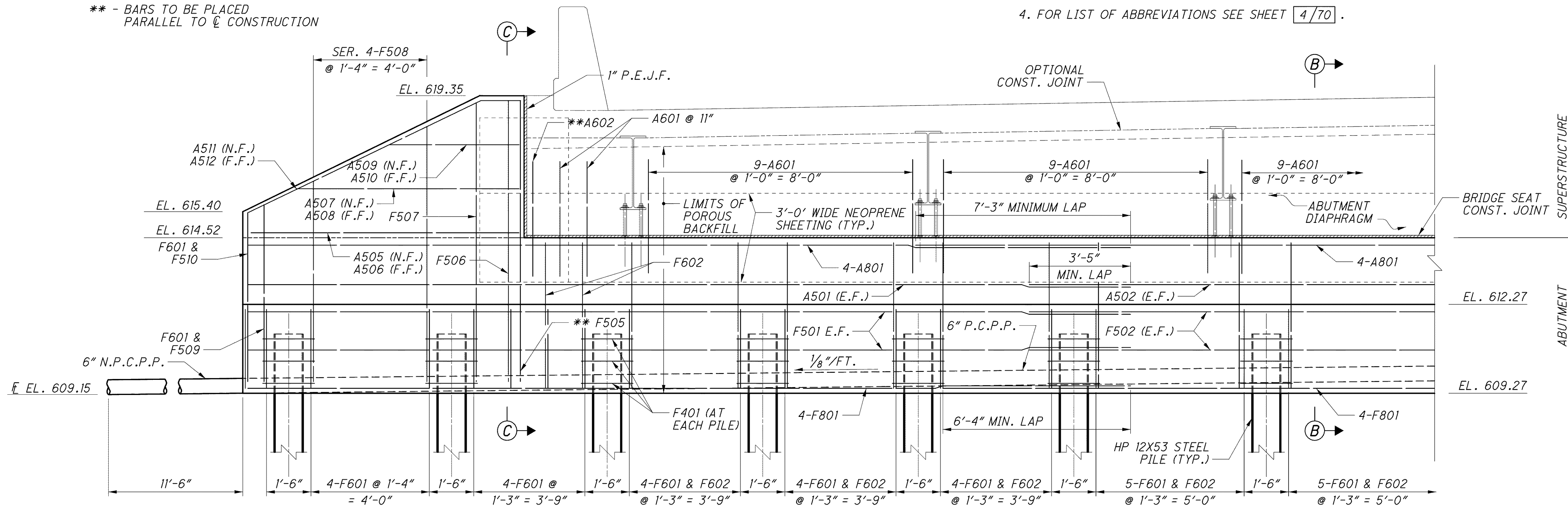
ELEVATION
