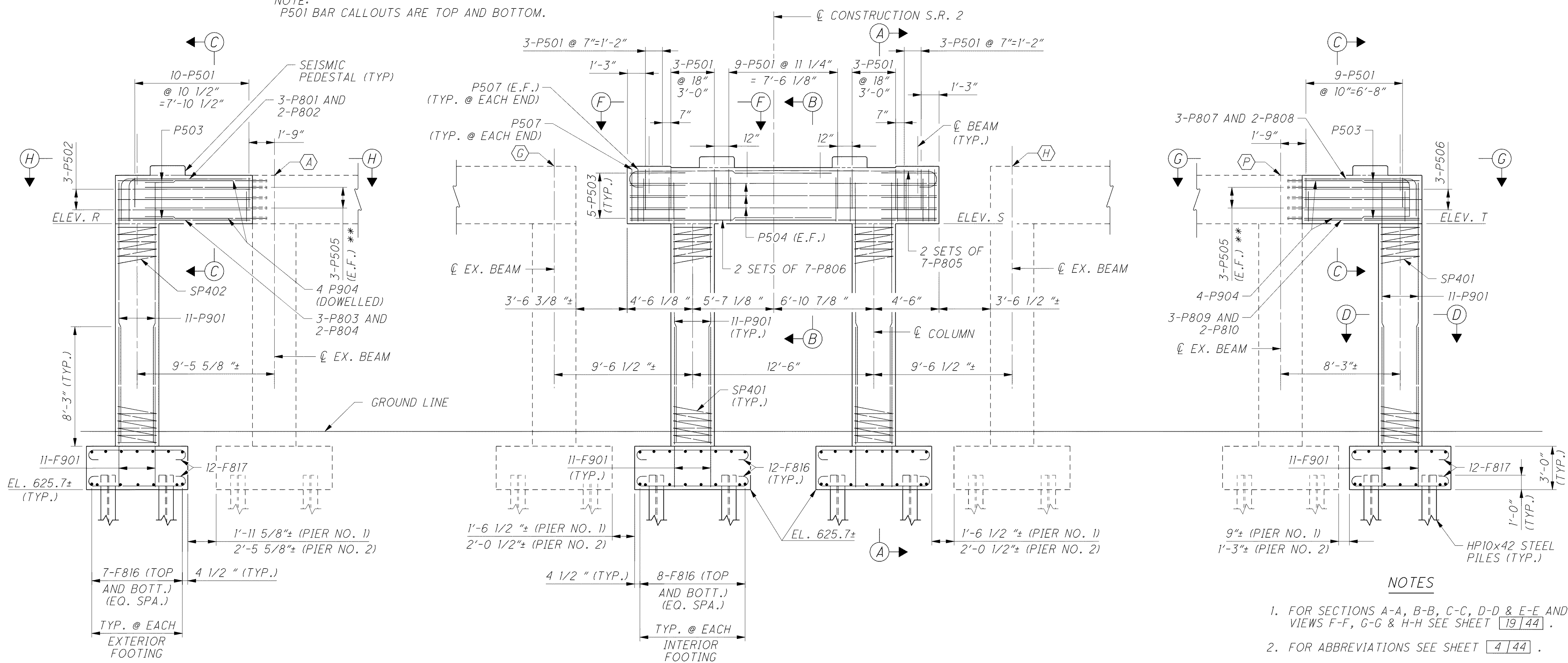
ELEVATION
