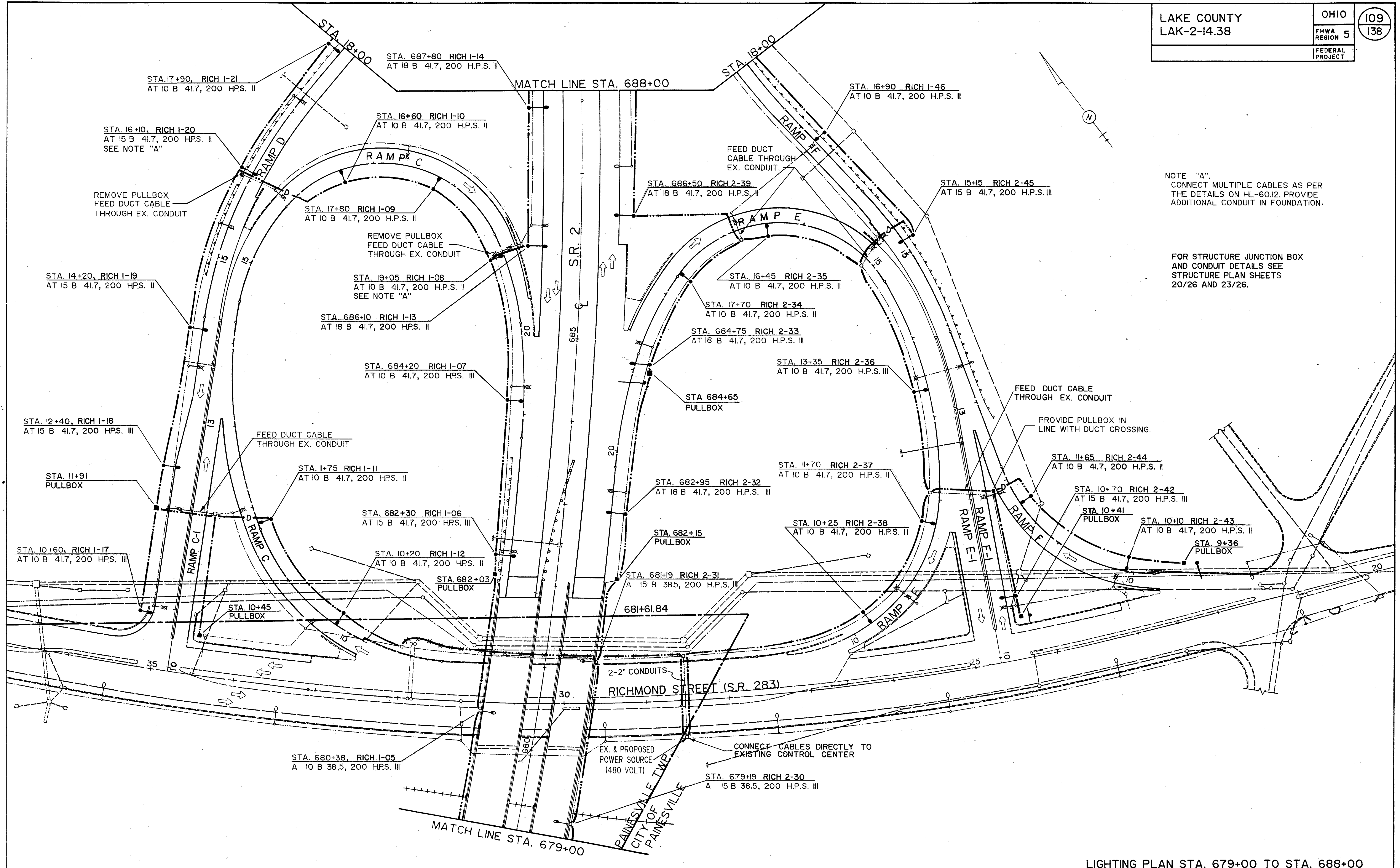
LIGHTING PLAN STA. 679+00 TO STA. 688+00
