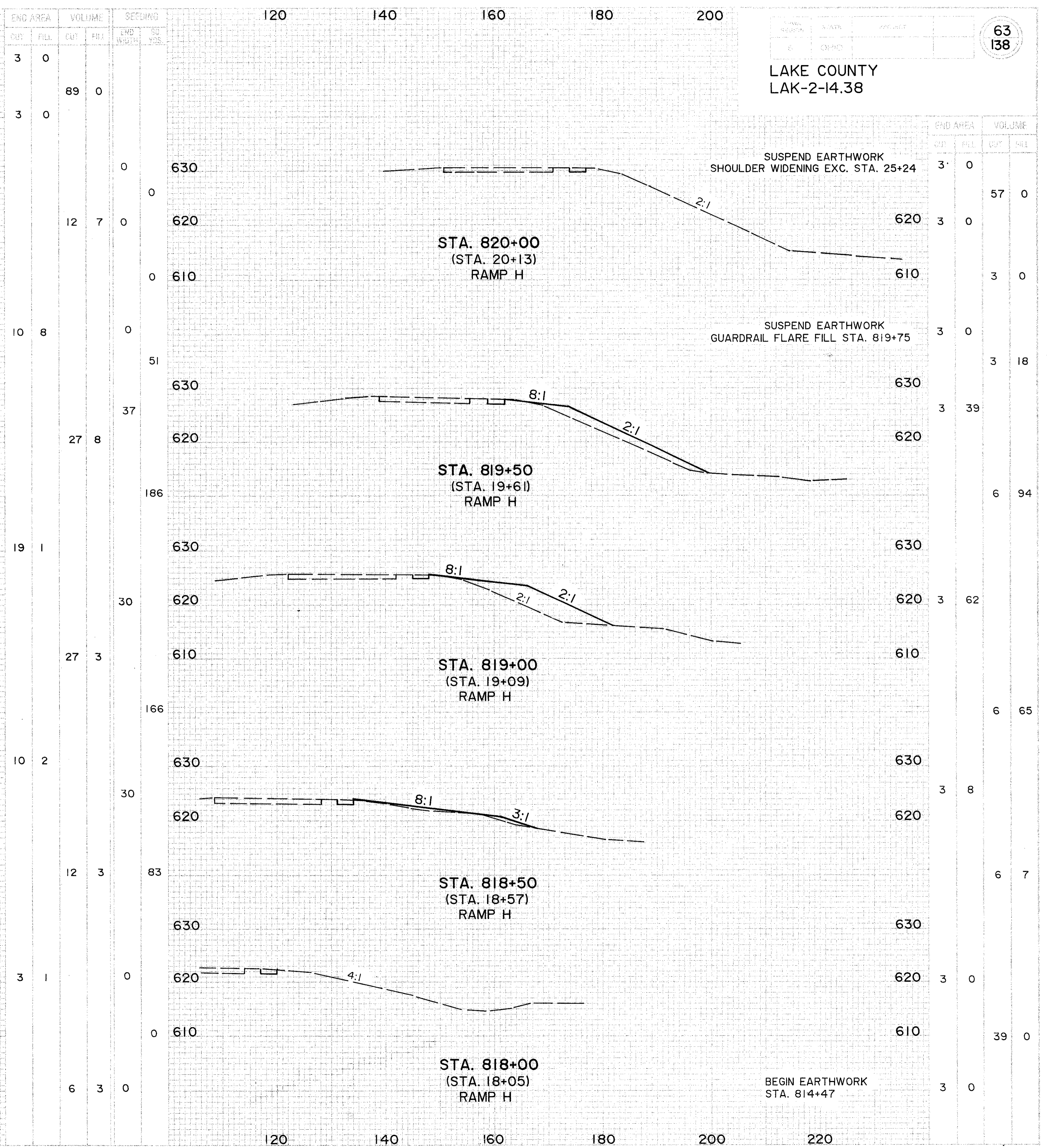
CROSS SECTIONS STA. 820+00 TO (RAMP G) STA. 13+00 (WB), (RAMP H) STA. 18+05 TO STA. 20+13 (EB)
