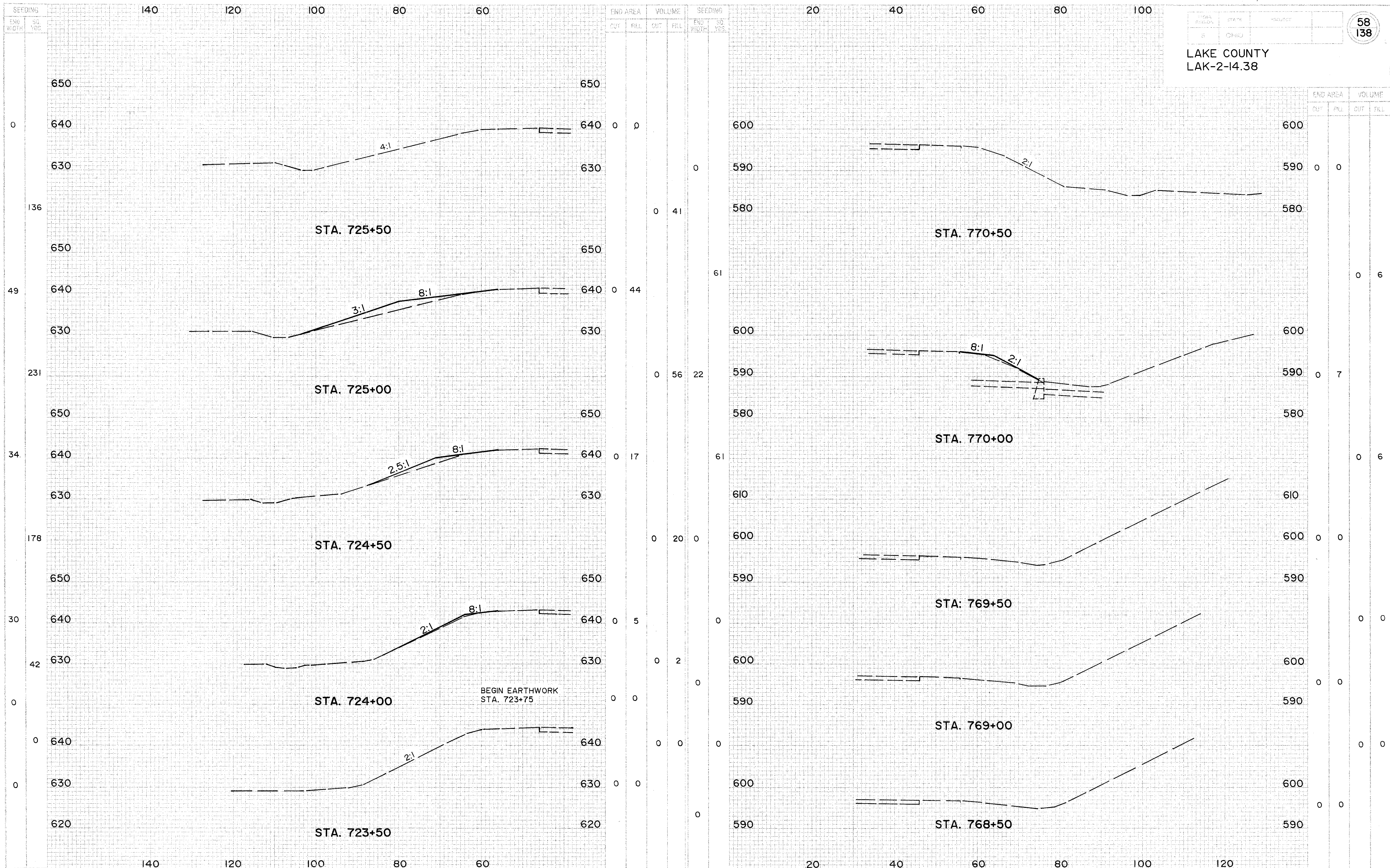
CROSS SECTIONS STA. 723+50 TO STA. 725+50 (WB), STA. 768+50 TO STA. 770+50 (EB)
