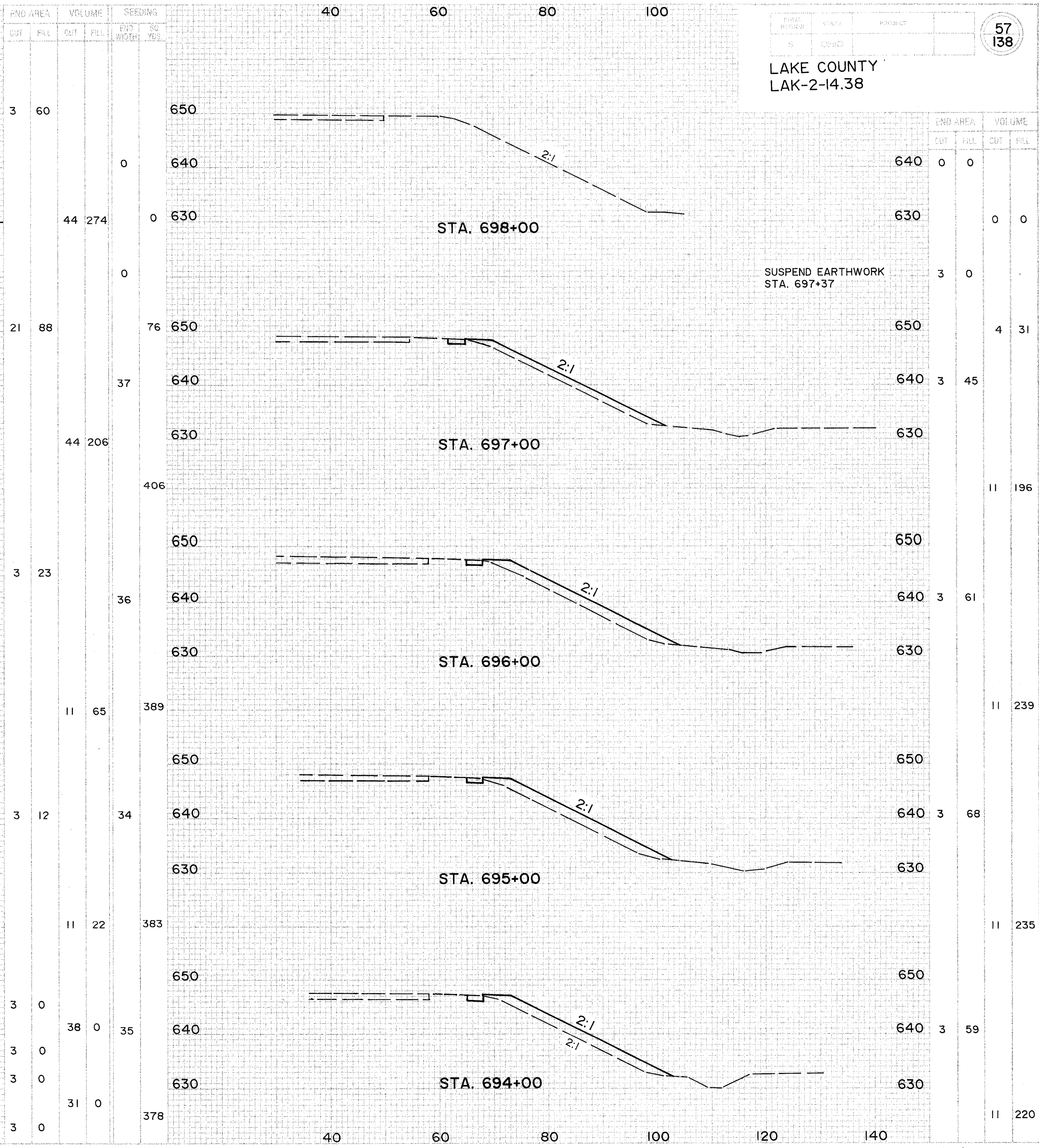
CROSS SECTIONS (RAMP F) STA. 19+00 TO (SR 2) STA. 698+00 (EB)
