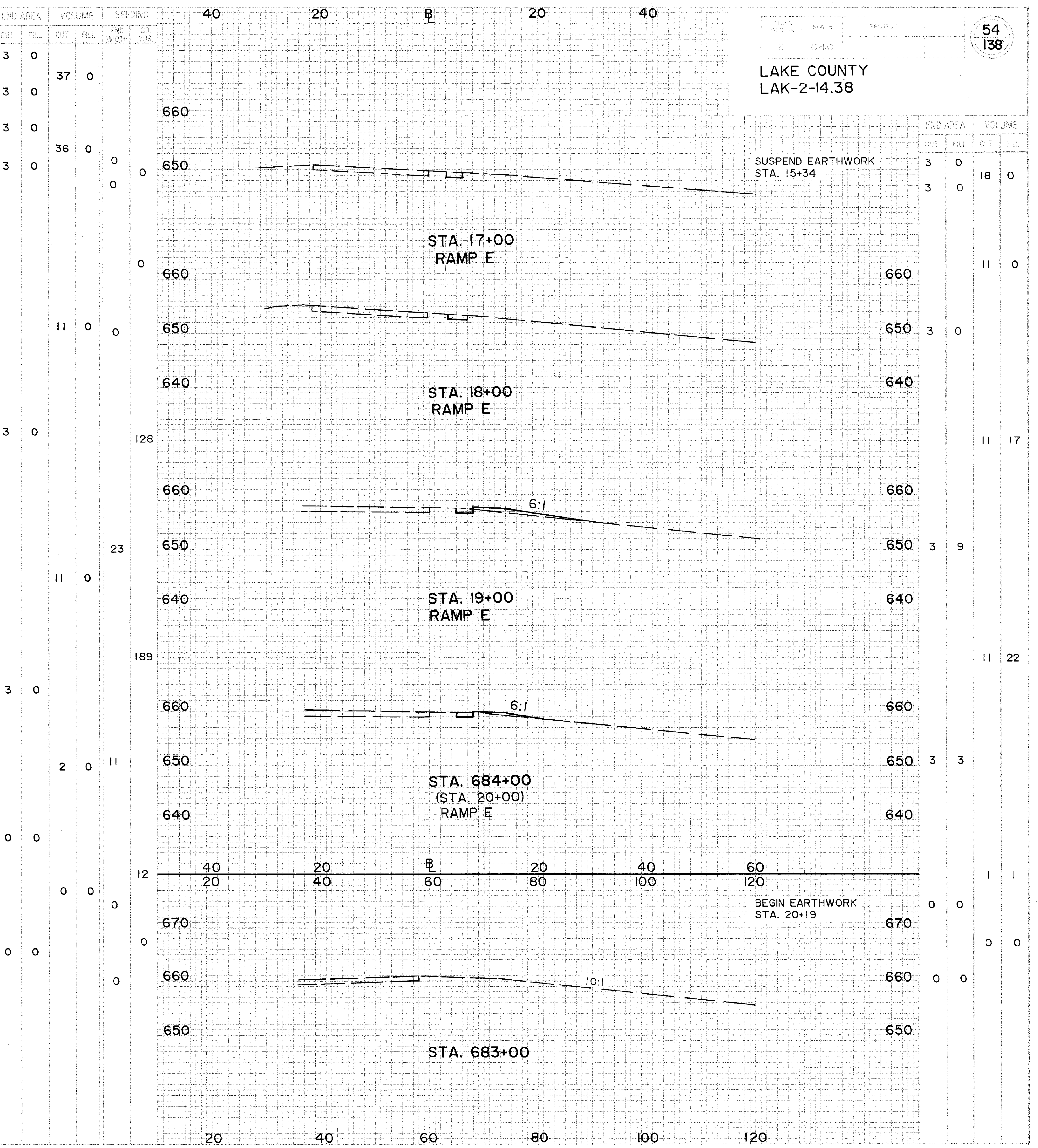
CROSS SECTIONS STA. 683+00 TO (RAMP C) STA. 19+00 (WB), STA. 683+00 TO (RAMP E) STA. 17+00 (EB)
