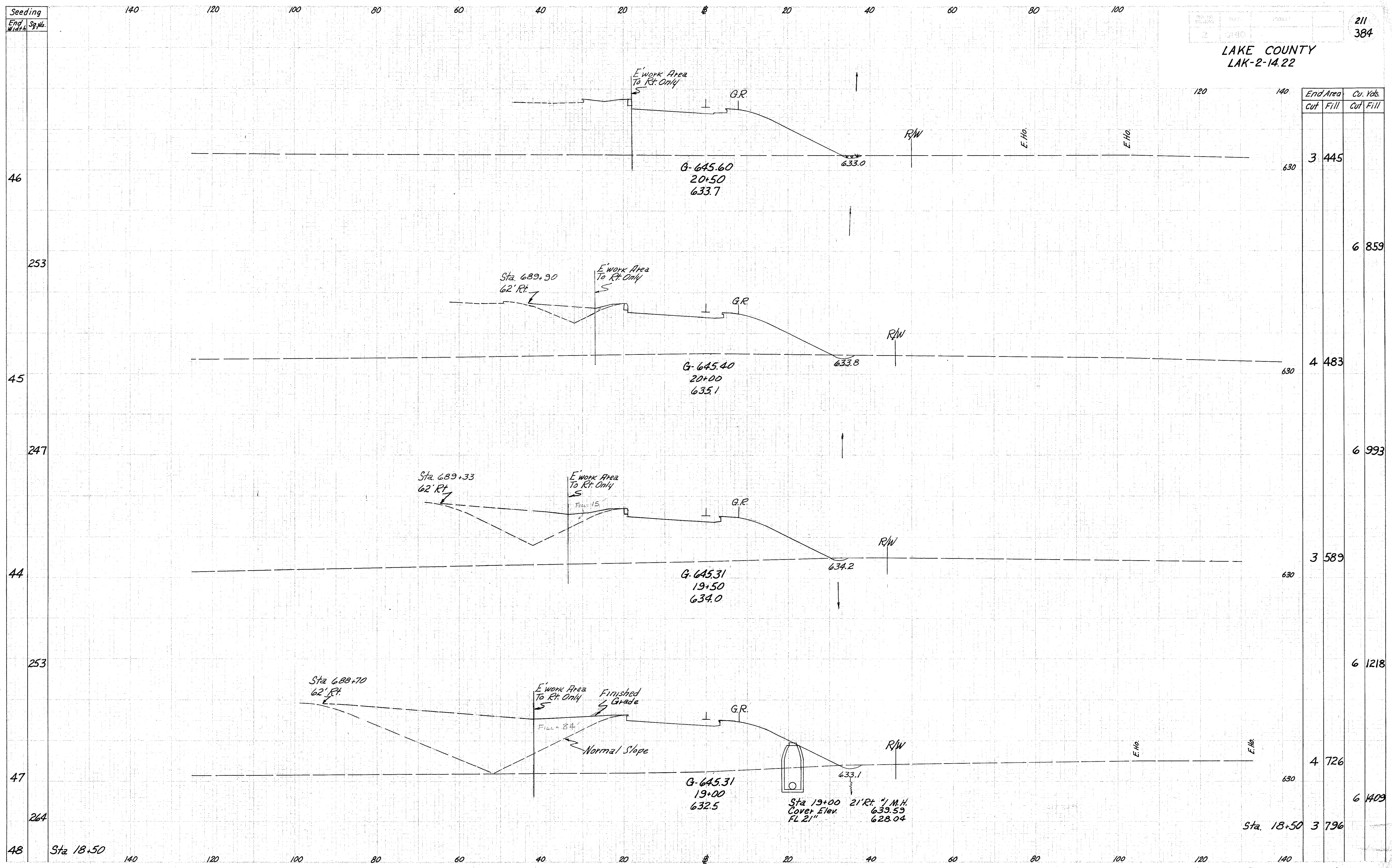
Ramp "FF" Sta. 19+00 to Sta. 20+50
