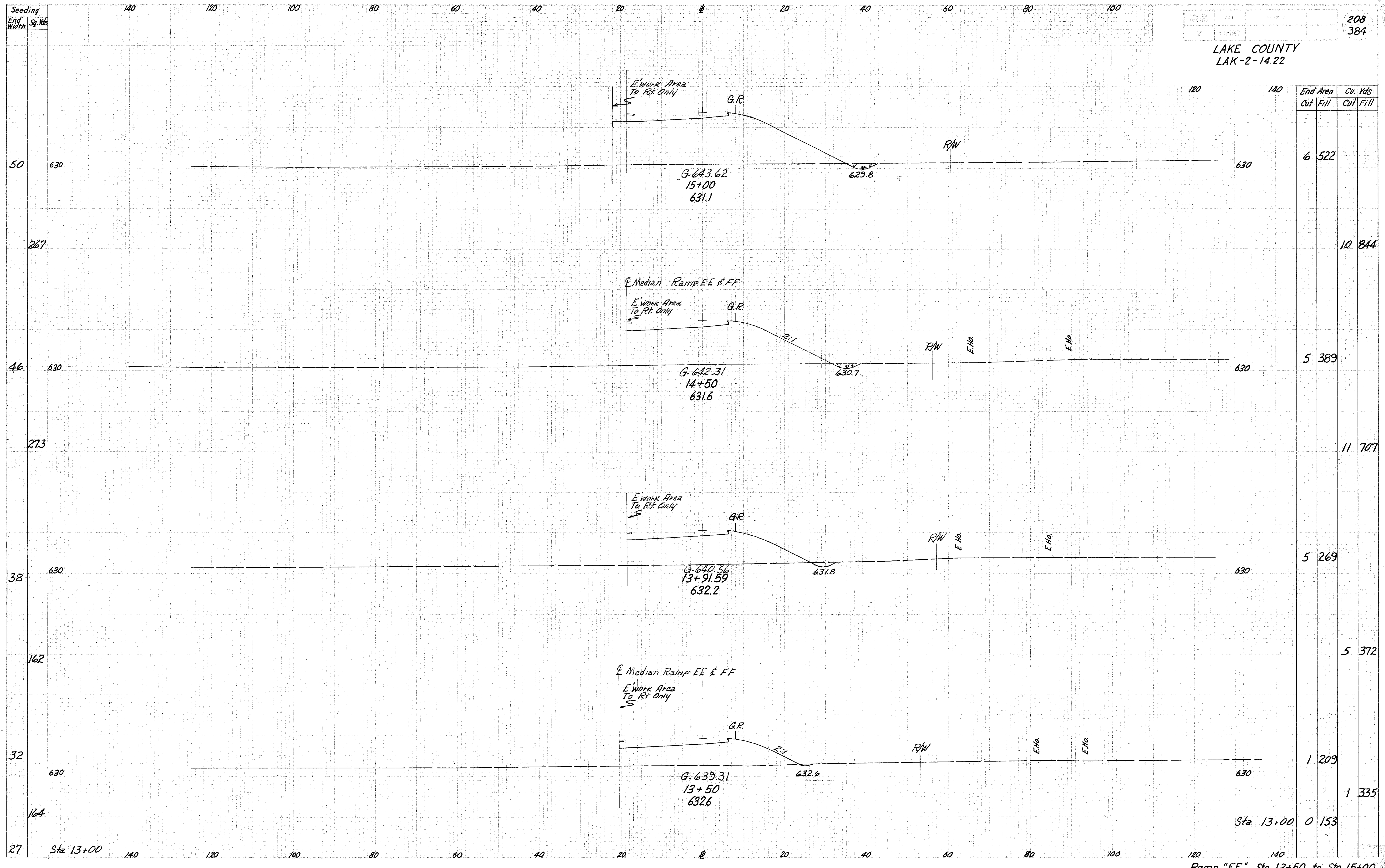
Ramp "FF" Sta. 13+50 to Sta. 15+00
