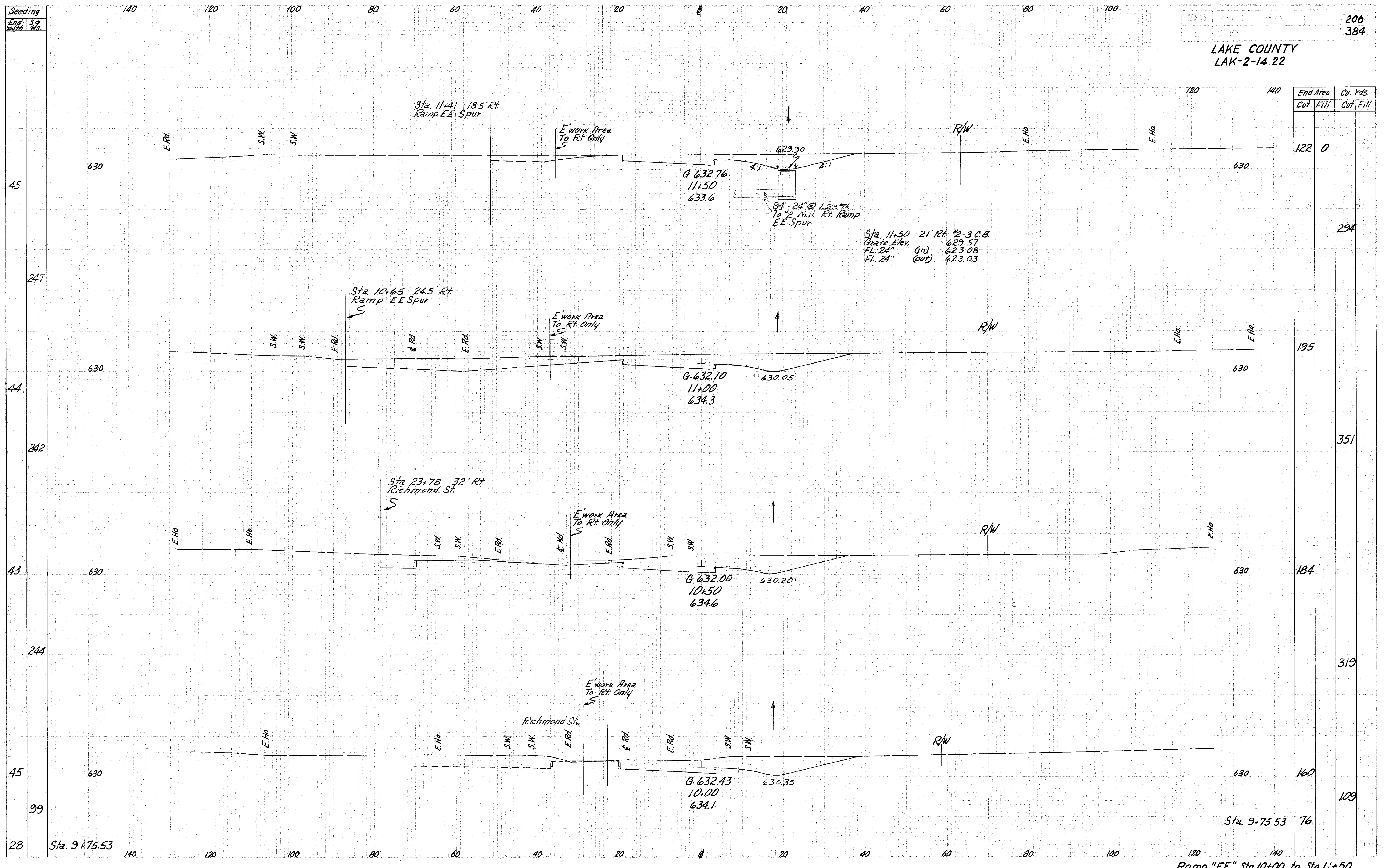
Ramp "FF" Sta. 10+00 to Sta. 11+50
