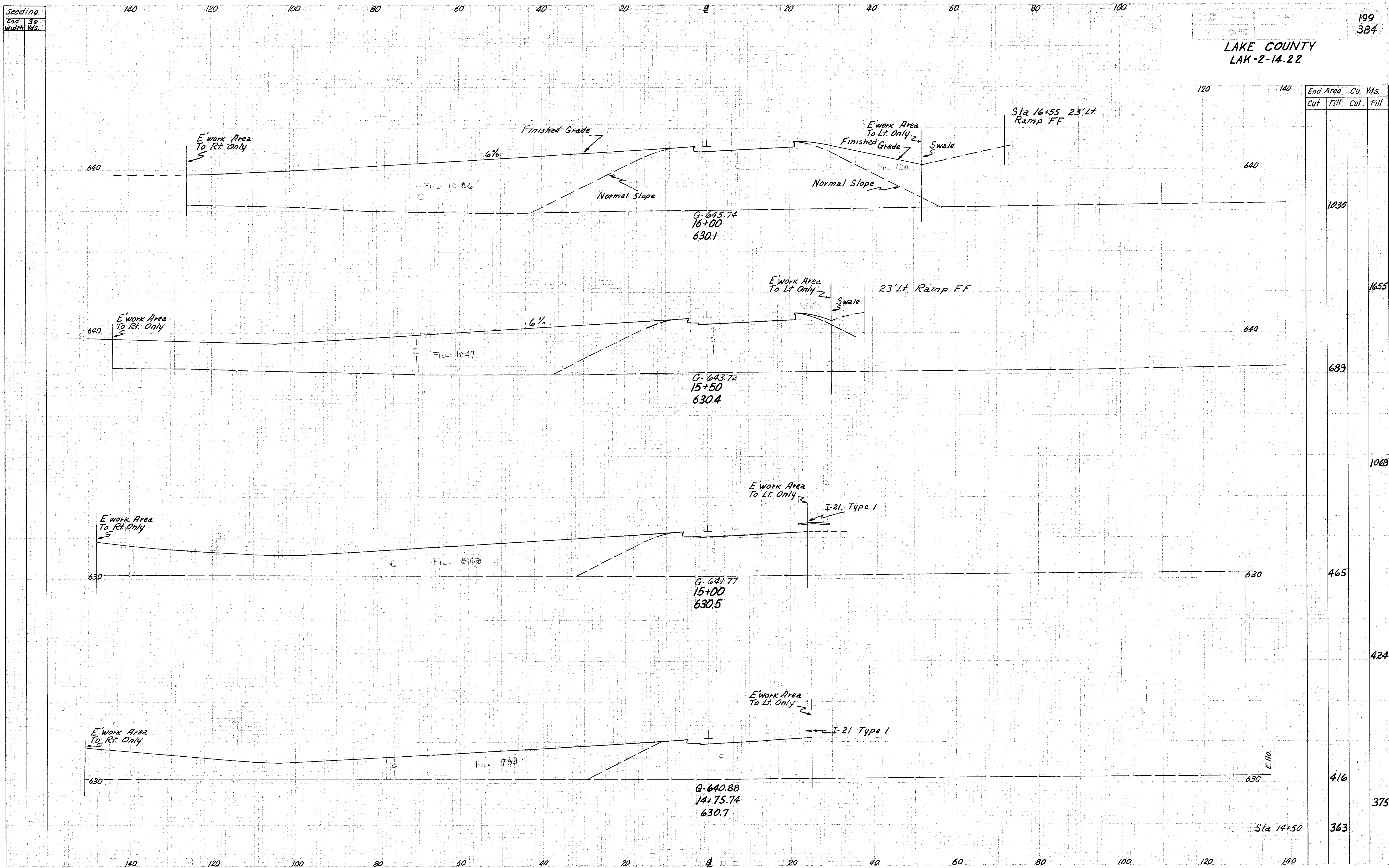
Ramp "EE" Sta. 14+75.74 to Sta. 16+00
