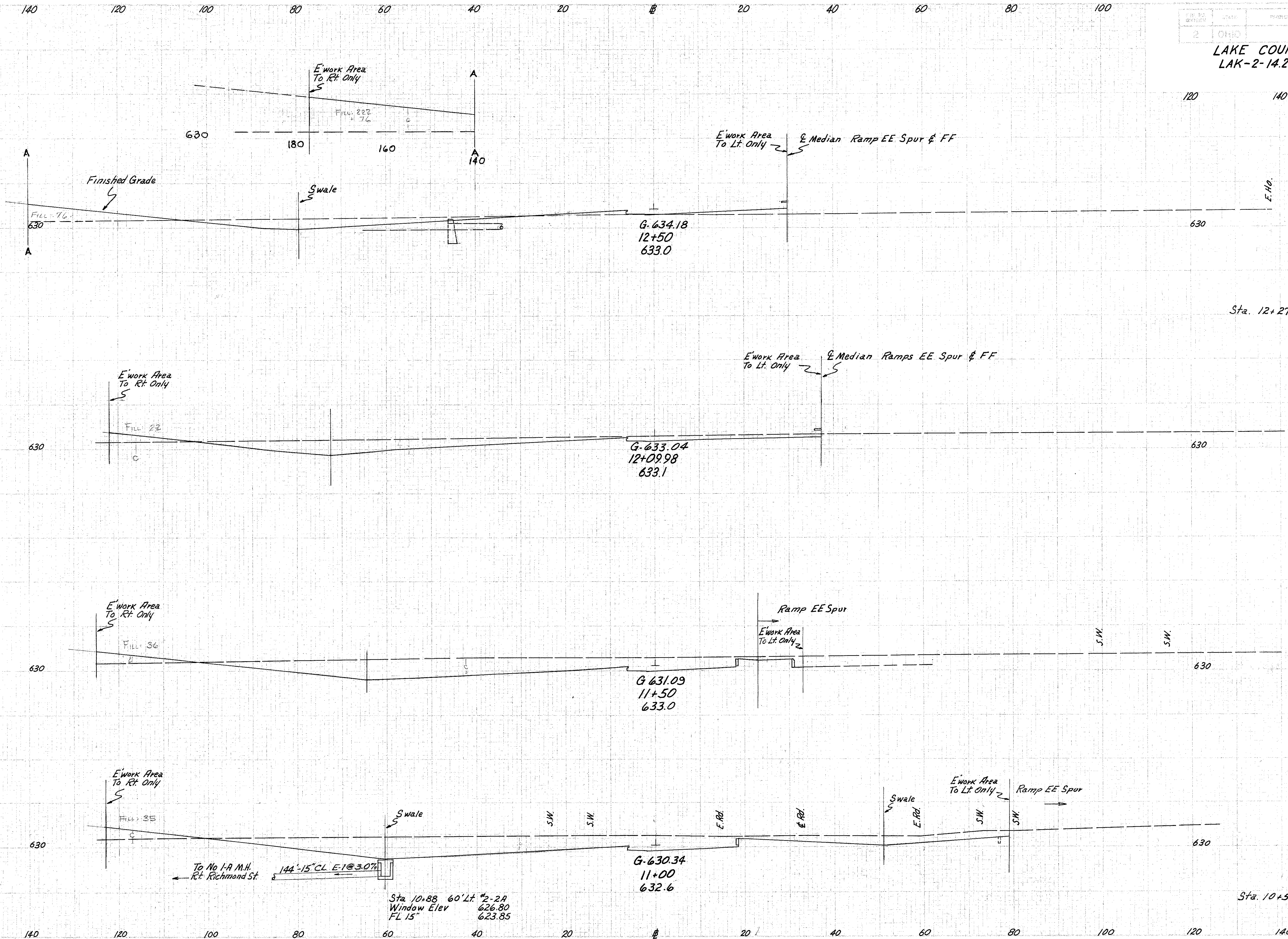
Ramp "EE" Sta. 11+00 to Sta. 12+50
