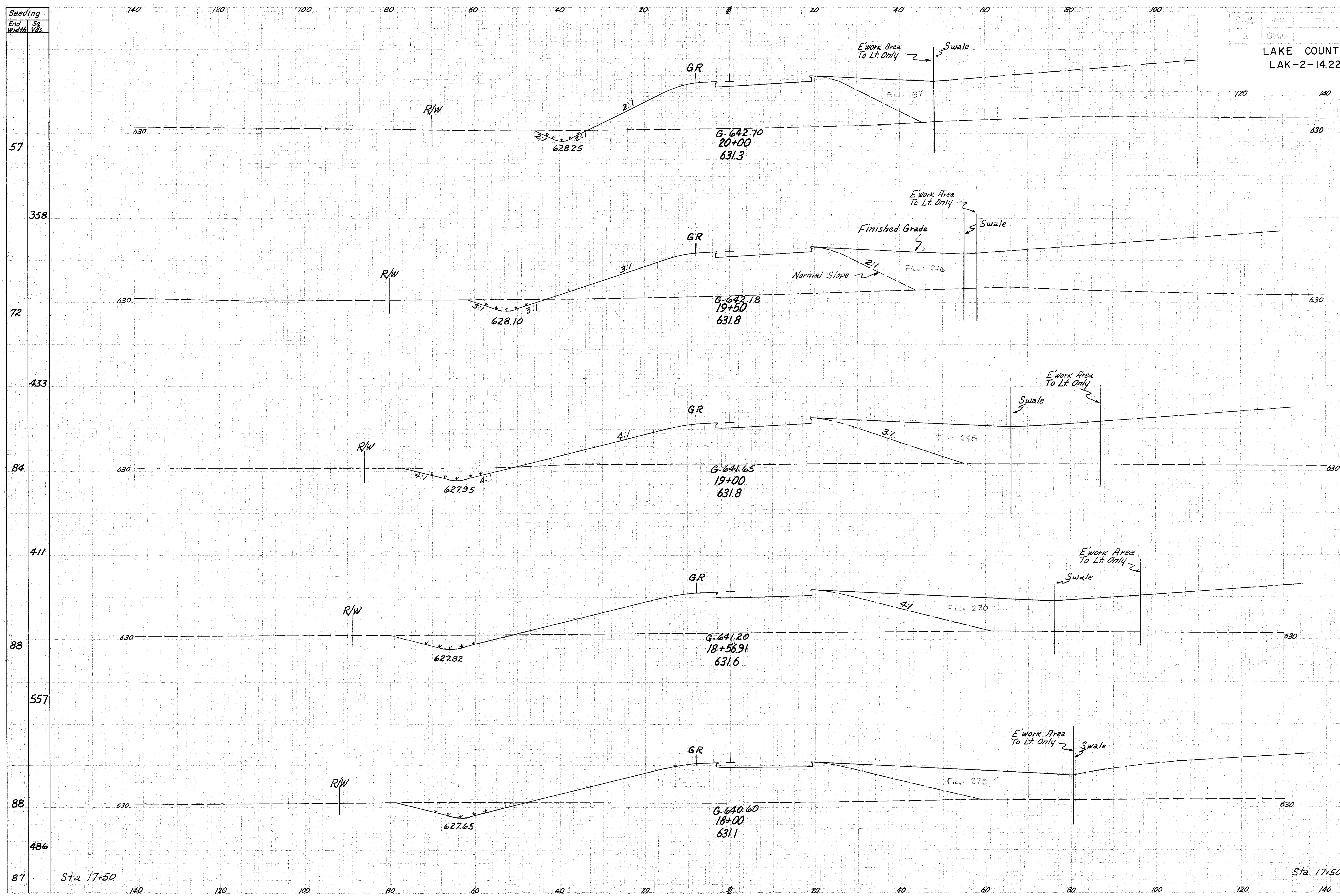
Ramp D-D Sta. 18+00 to Sta. 20+00
