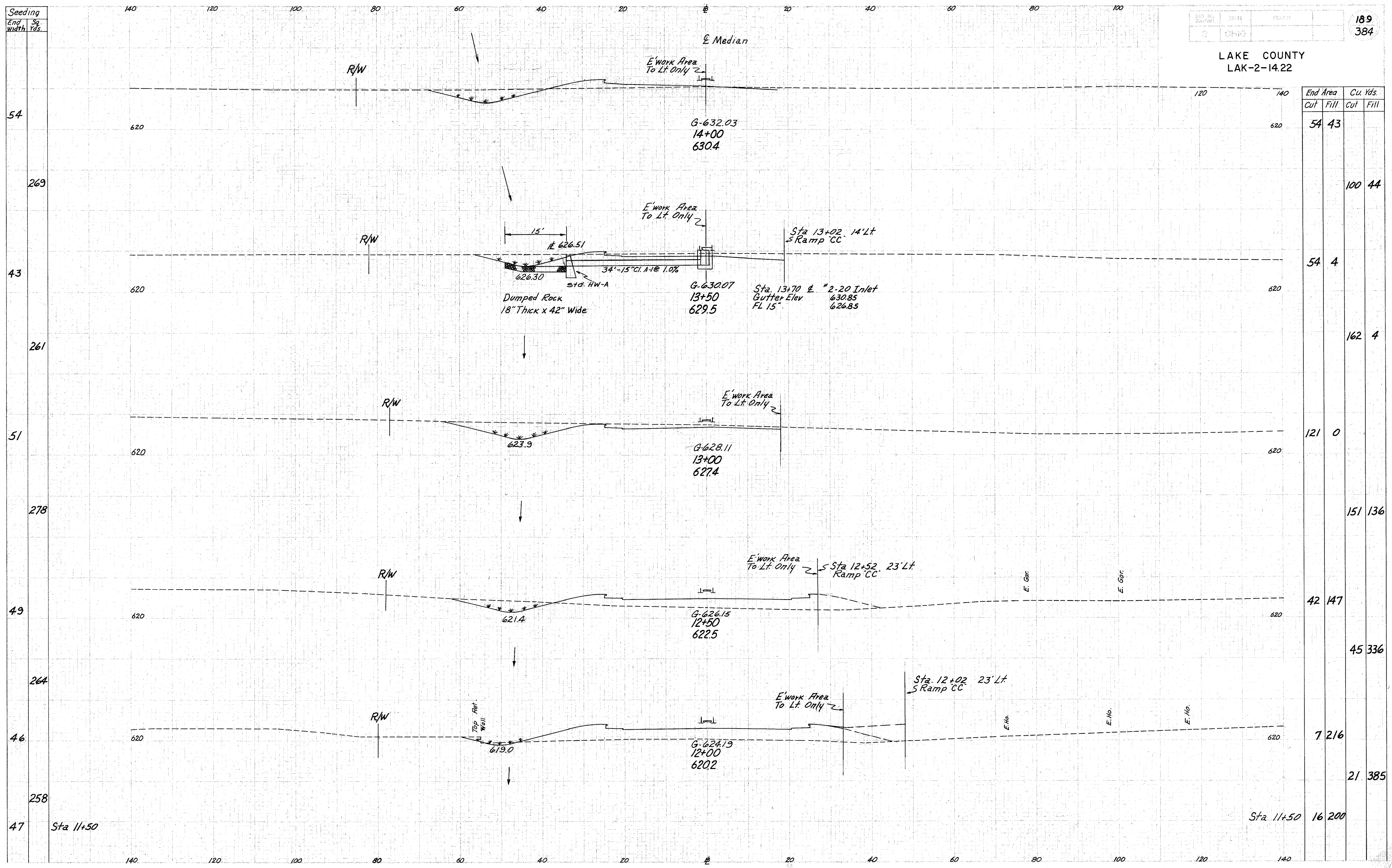
Ramp D-D Sta 12+00 to Sta 14+00
