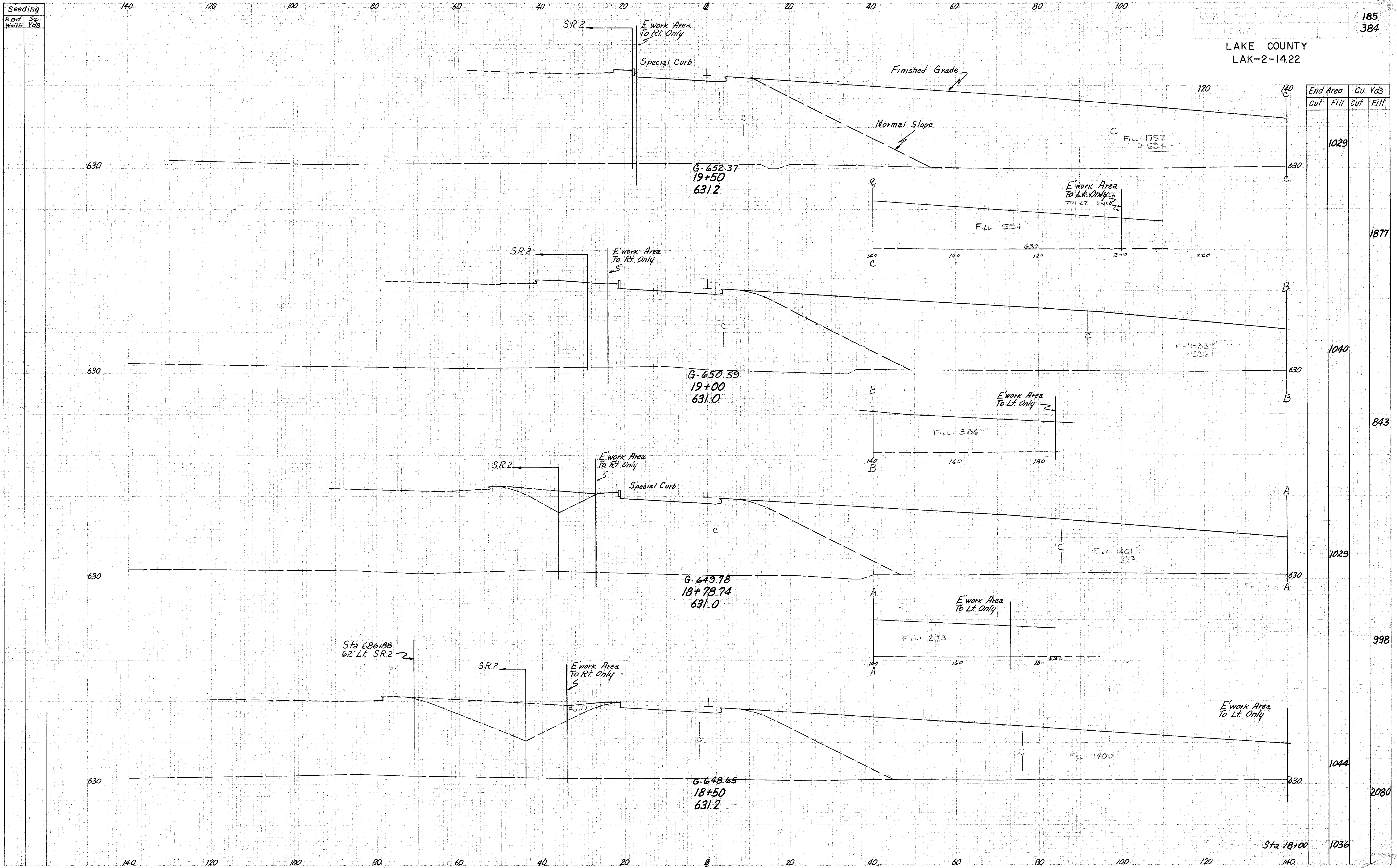
Ramp C-C Sta. 18+50 to Sta. 19+50
